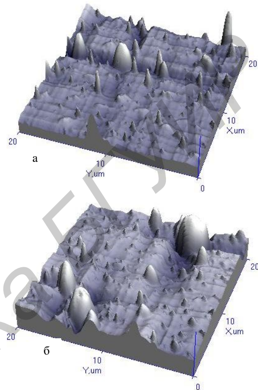
Рис. 5. 3D - изображения топографии поверхностей пленки Al (99.995%) (а), пленки сплава Al-1.0 ат.% Cr (б), нанесенной на стекло методом ОПАСИ при ускоряющем напряжении 3 кВ при силе ионного тока ~ 100 мкА за 10 часов.
