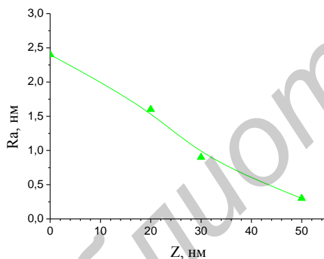
Рис. 3. Зависимость шероховатости поверхности Mo пленки от толщины осажденной пленки.
