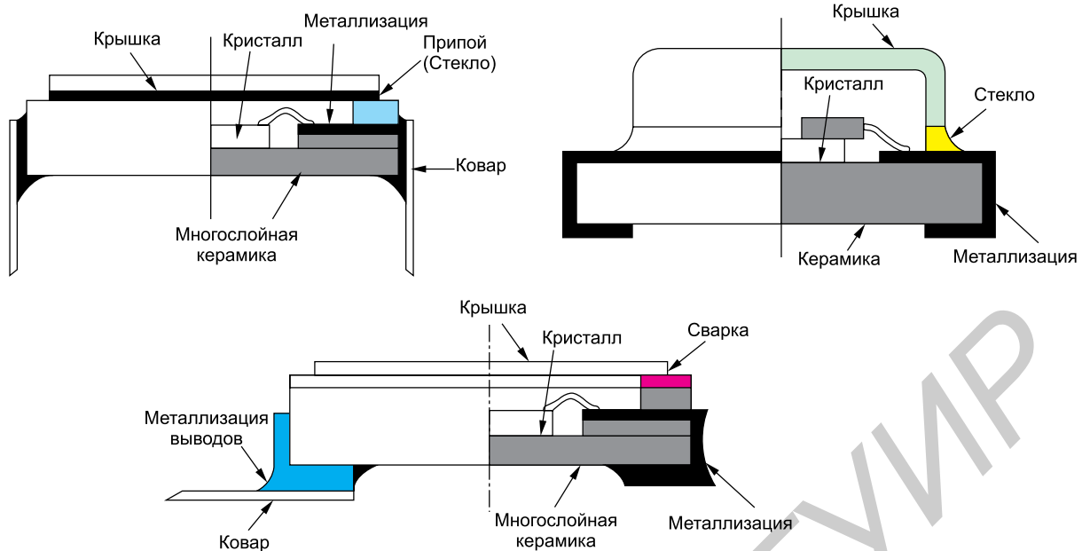
Рис. 2. Способы герметизации корпусов ИС
