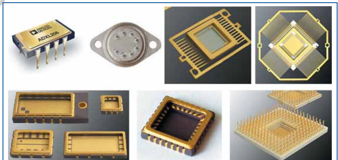
Рис. 1. Современные герметичные корпуса для ИС
