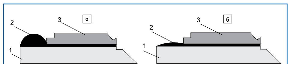
Рис. 4. Форма паяного шва: а) с прижатием крышки; б) без прижатия в процессе герметизации (1 — основание корпуса; 2 — галтель припоя; 3 — крышка)
