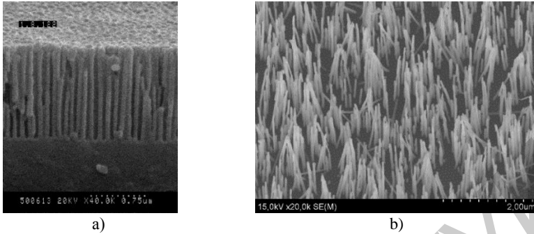
Рис. 4. Электронно-микроскопические снимки матриц АОА на кремниевой подложке для формирования матрицы нанопроводов (а) и массива нанопроводов InSb на подложке после селективного удаления матрицы АОА (б).
