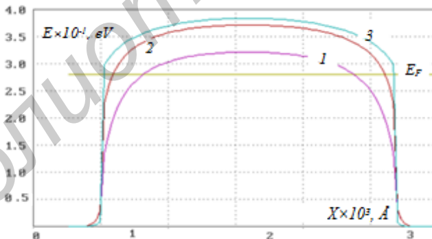
Рис. 2. Потенциальные рельефы для электронов в нанопроводе при нулевом приложенном напряжении комнатной температуре и различных поперечных размерах проводящего канала L_{\perp} : 1 — L_{\perp} = L_{dq}/2 ; 2 — L_{\perp} = L_{dq}/3 ; 3 — L_{\perp} = L_{dq}/4 . L_{dq} — длина размерного квантования [3].
