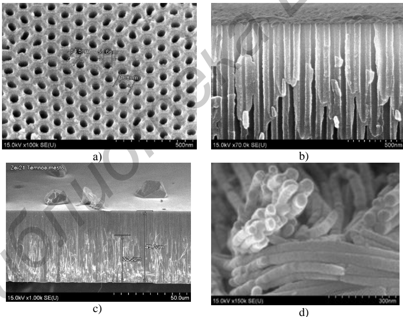
Рис. 5. Электронно-микроскопические снимки поверхности (а) и поперечного сечения матриц АОА (б), сечения подложки с осажденными InSb нанопроводами (с), и нанопроводов InSb после селективного удаления подложки АОА (д).
