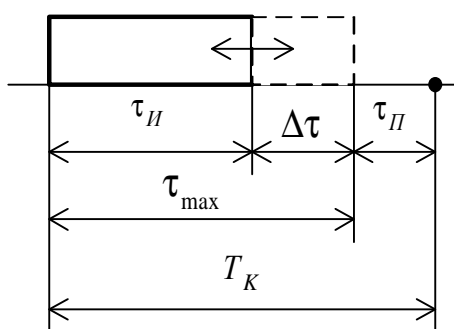
Рис. 1.13. Разметка канального интервала при ШИМ
