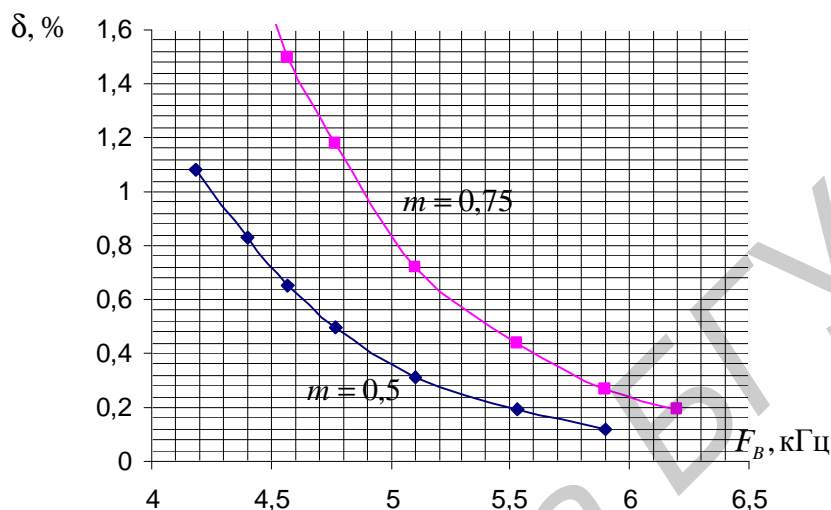
Рис. 1.18. Зависимость ошибки в системе с АИМ от полосы пропускания видеотракта
