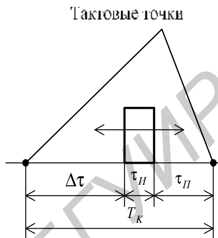
Рис. 1.14. Разметка канального интервала при ФИМ
