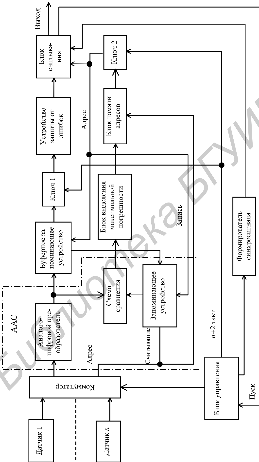
Рис. 1.41. Структурная схема КТ телеметрической системы с адаптивной коммутацией
