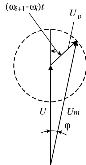
Рис. 1.7. Векторная диа-
