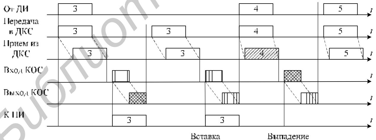
Рис. 4.5. Появление сдвига при работе системы ПДС с РОС-ОЖ
