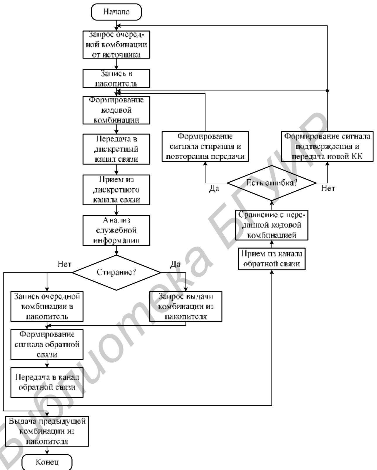
Рис. 4.7. Схема алгоритма работы системы с ИОС
