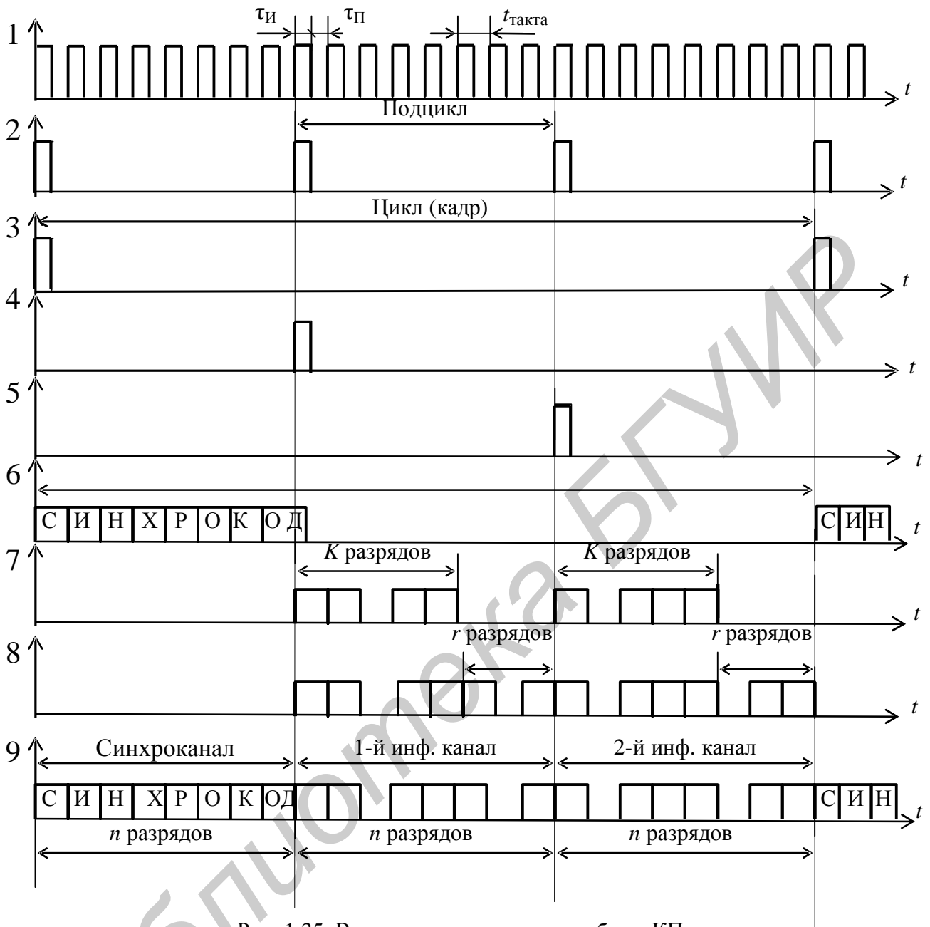
Рис. 1.35. Временные диаграммы работы КИП
