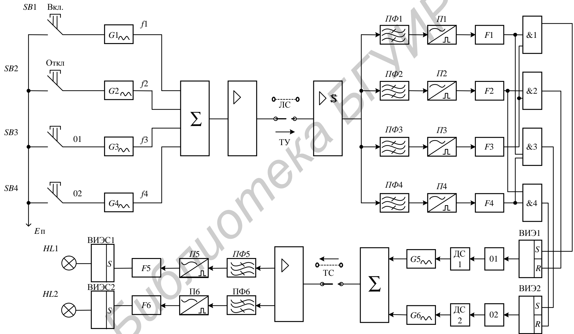
Рис. 2.2. Функциональная схема устройства ТУ-ТС с частотным методом избираня и сигнализацией по методу «светлого» щита
