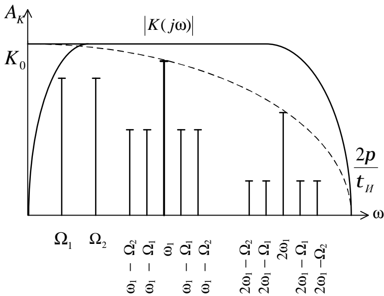
Рис. 1.15. АЧХ группового тракта
