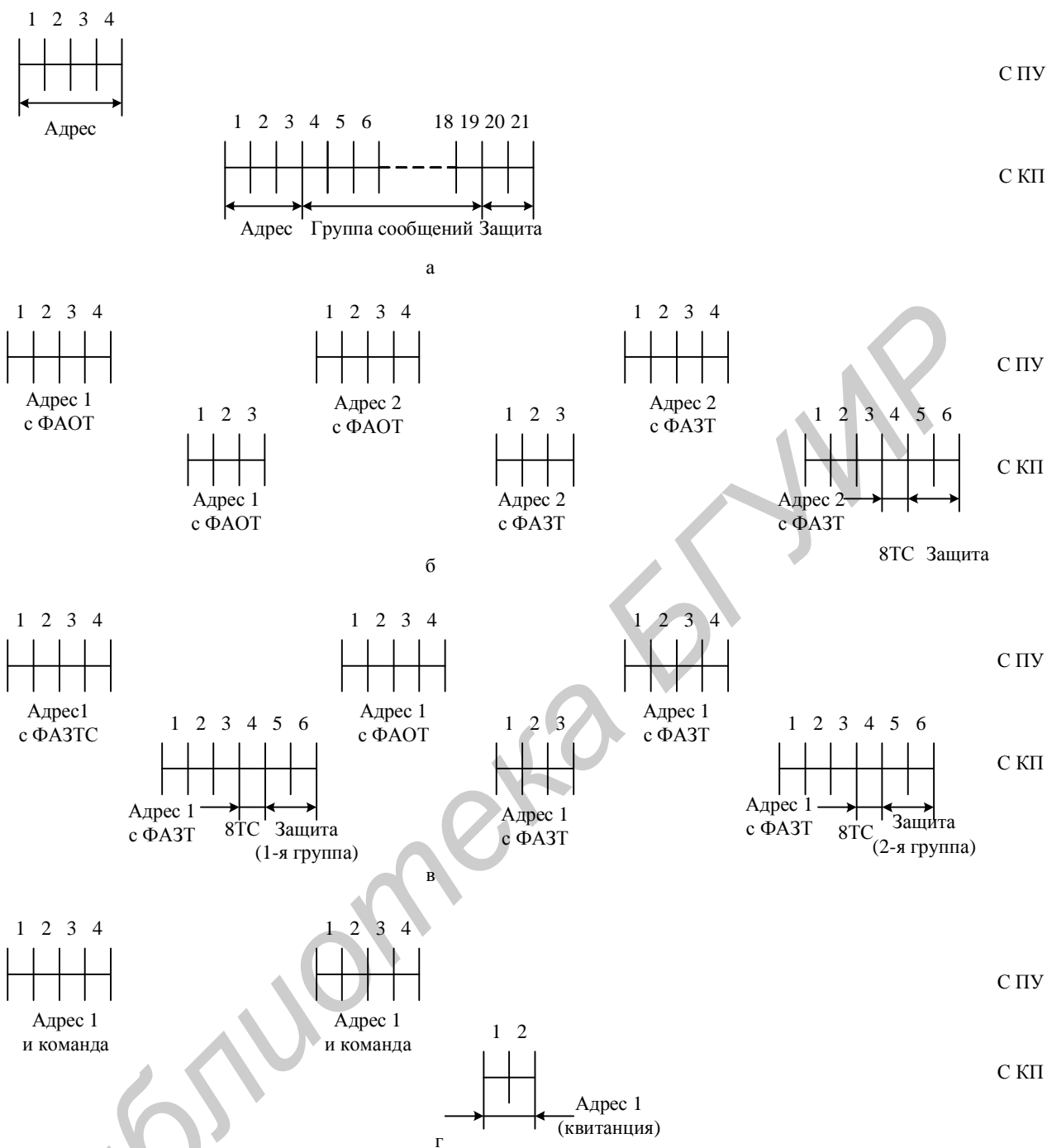
Рис. 6.11. Диаграмма обмена сигналами между ПУ и КП ТМ-120-1
