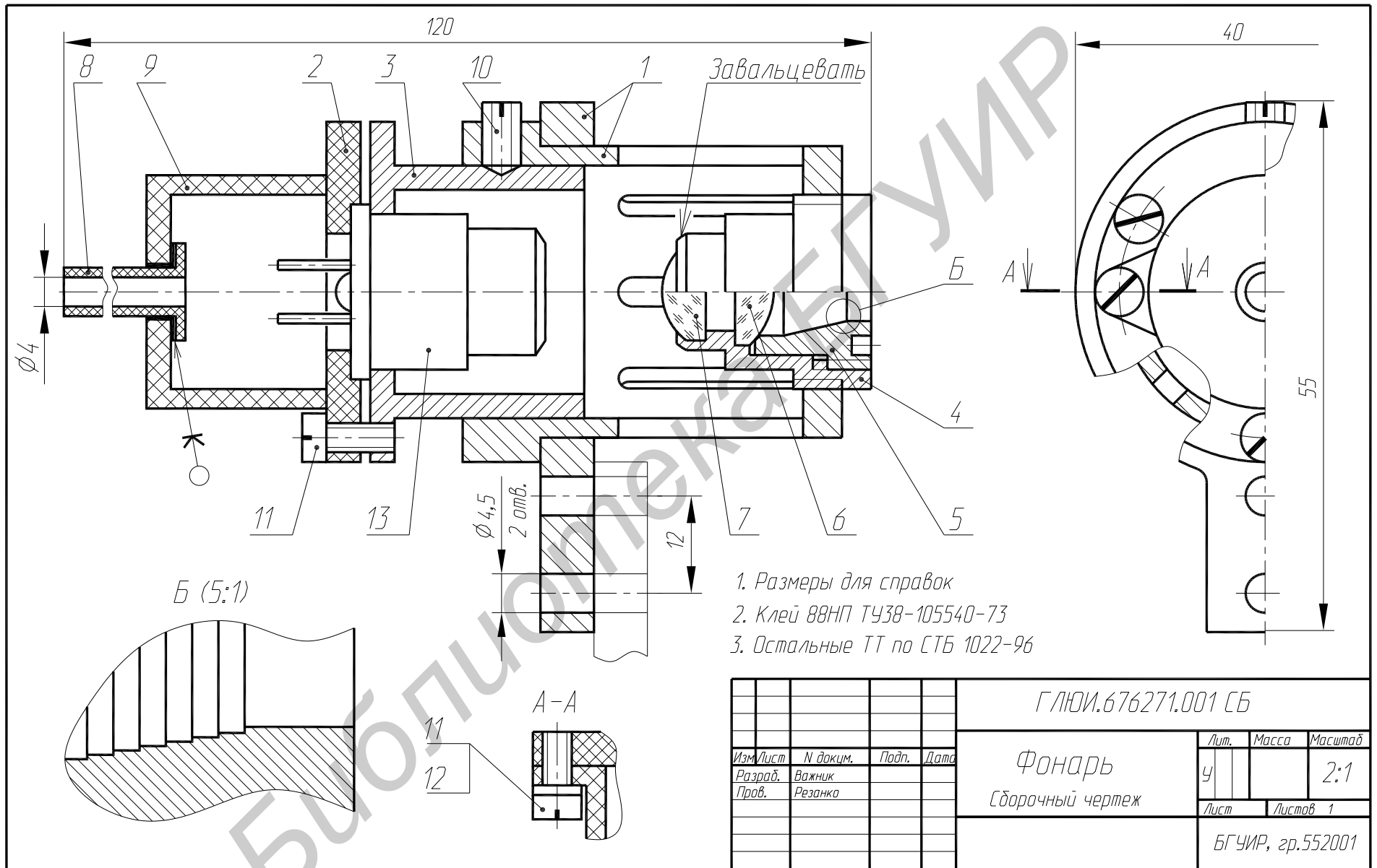
Рис. 1. Пример сборочного чертежа
