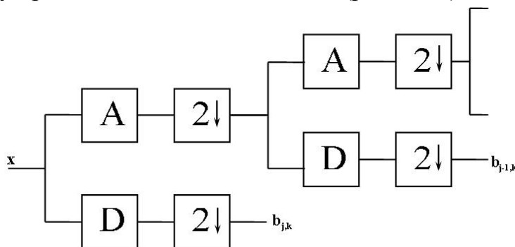
Рис. 4.10. БВП. Логарифмическое дерево банков фильтров
