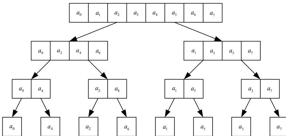
Рис. 1.7. Дерево рекурсий для 8 элементов
