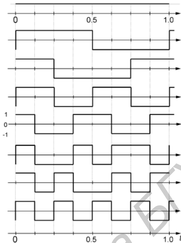
Рис. 3.2. Первые восемь функций Уолша
