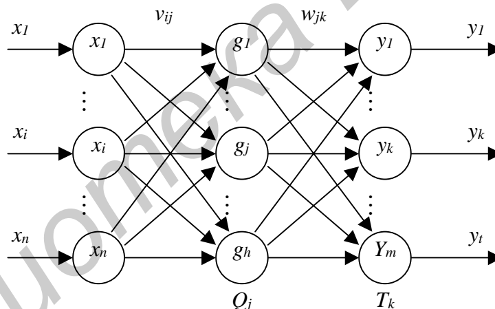
Рис. 2.1. Многослойный персептрон
