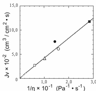
Рис. 1. Зависимость потоков чистых растворителей от обратной вязкости: □ – этанол; ● – бензол; Δ – вода; ○ – метанол; ■ – ацетон; Jv – поток жидкости ( \text{см}^3 / \text{см}^2 \cdot \text{сек} ); P_a = P_1 - P_2 – разность давлений по обе стороны мембраны; \eta – вязкость ( P_a \cdot \text{сек} )
