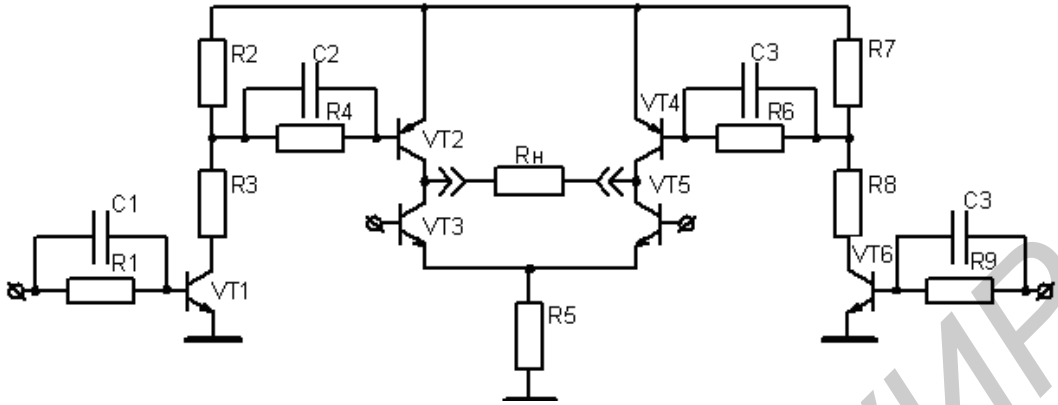
Рисунок 2.6 – Электрическая принципиальная схема каскада блока ЭА
