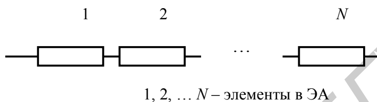
Рисунок 2.5 – Схема (модель) соединения элементов в ЭА с точки зрения надёжности
