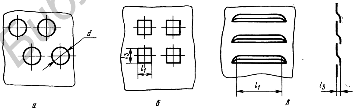
Рисунок 2.4 – Конфигурация перфорационных отверстий
