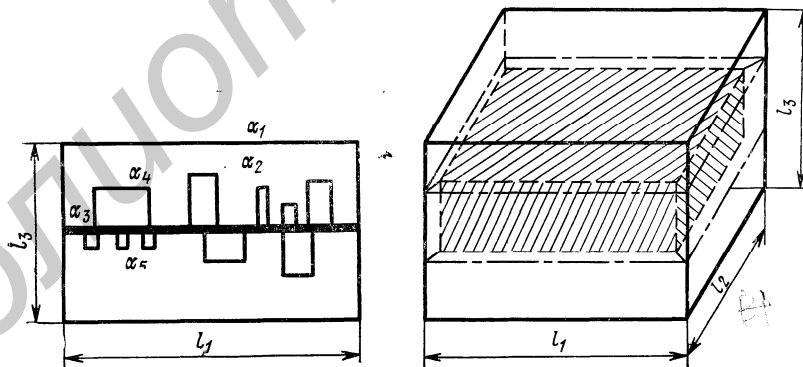
Рисунок 2.2 – Схематическое изображение блока ЭА в герметичном корпусе и его физическая тепловая модель
