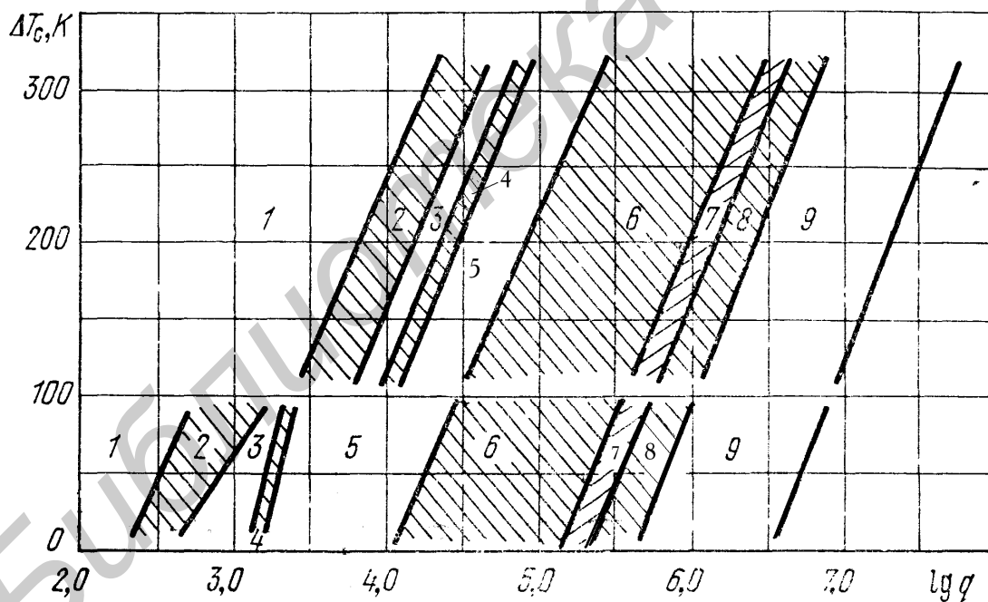
Рисунок 2.1 – Выбор способа охлаждения ЭА
