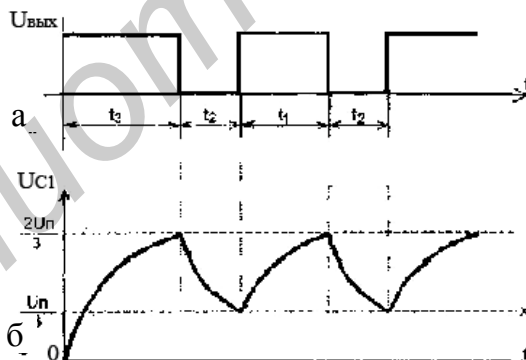
Рисунок 5.4 – Форма выходного сигнала и напряжения на конденсаторе
