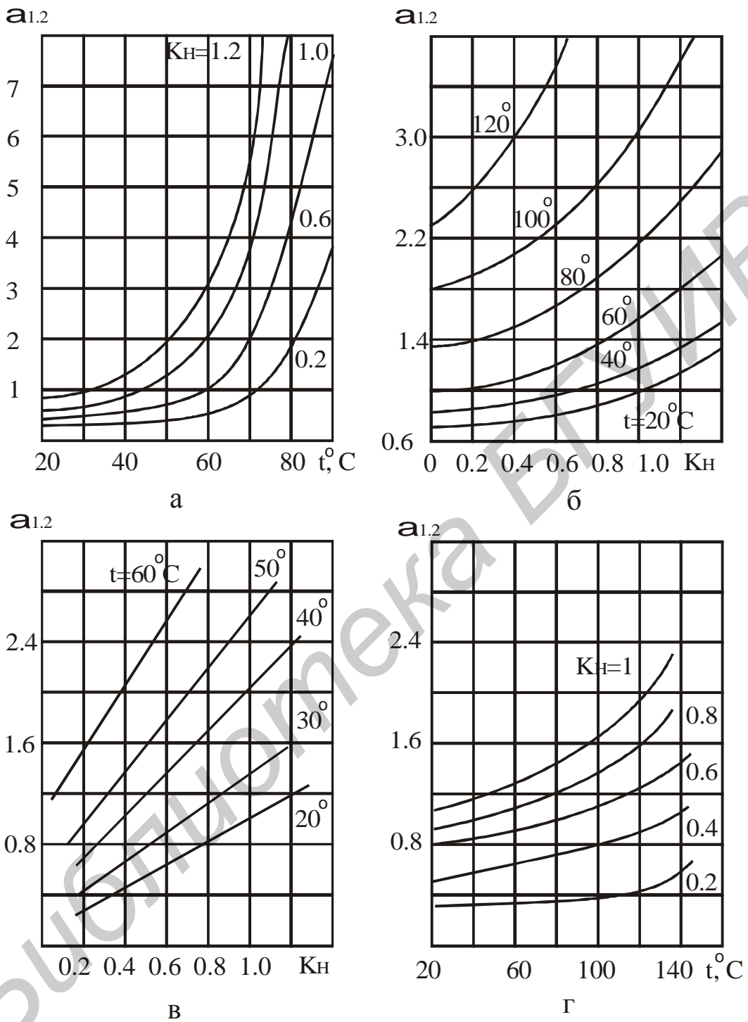
а – для германиевых диодов; б – для кремниевых диодов; в – для германиевых транзисторов; г – для кремниевых транзисторов Рисунок Г.3 – Обобщенные зависимости поправочного коэффициента \alpha_{1,2} от температуры и коэффициента нагрузки
