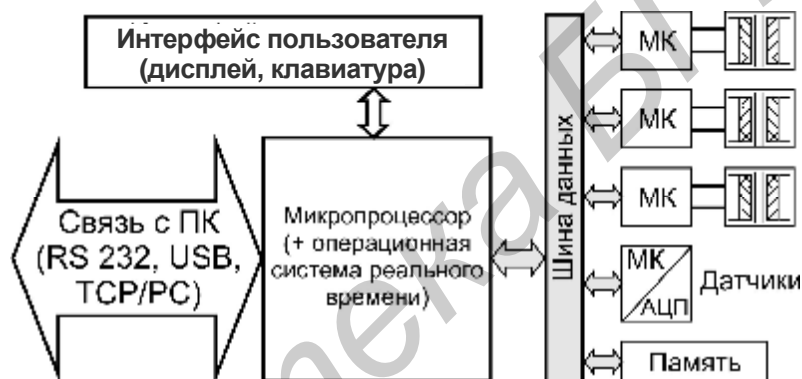
Рисунок 4.8 – Многопроцессорная терапевтическая система
