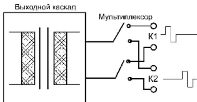
Рисунок 4.6 – Многоканальное устройство с мультиплексором
