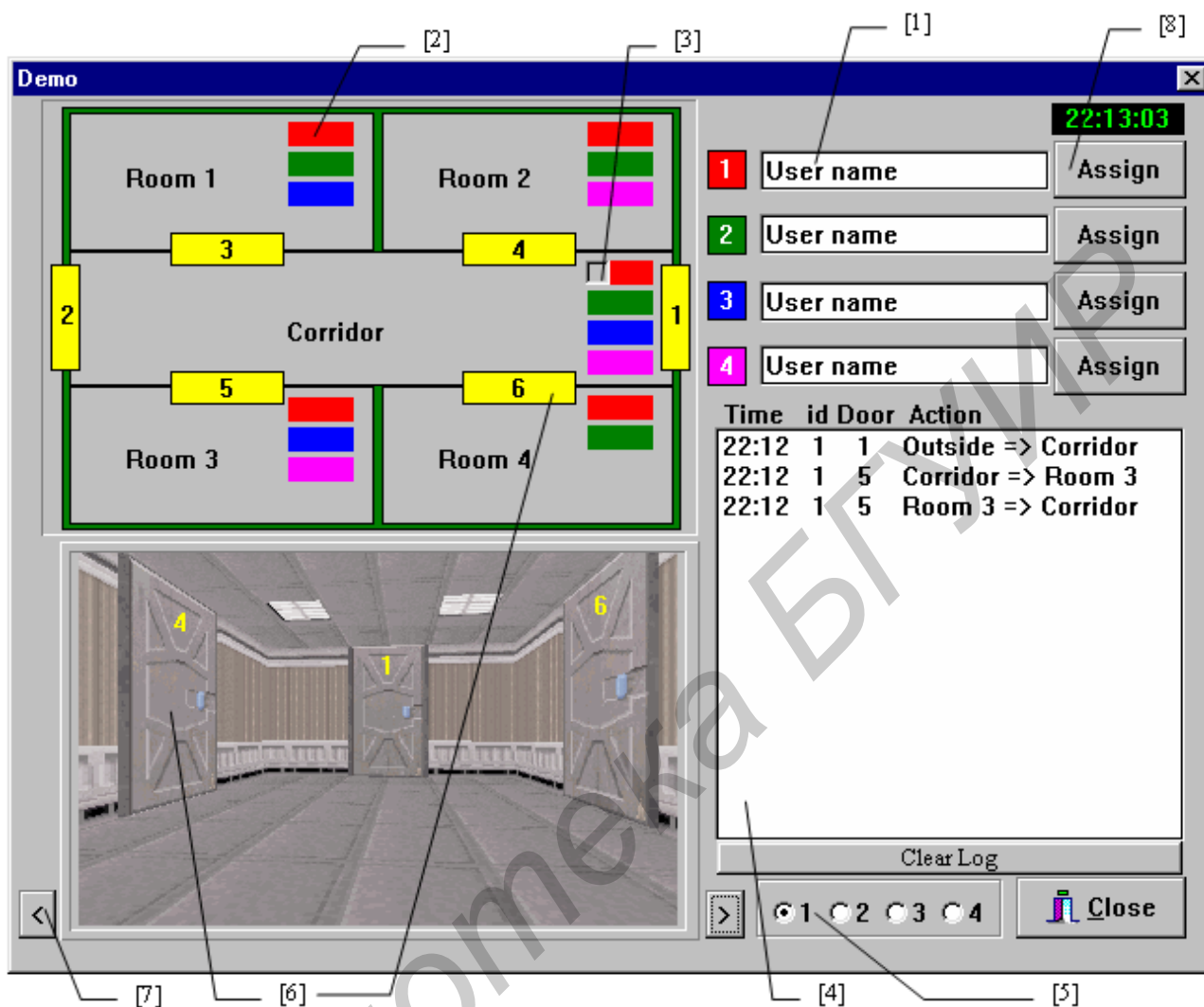
Рис. 4.4. Интерфейс программы Demo.exe
