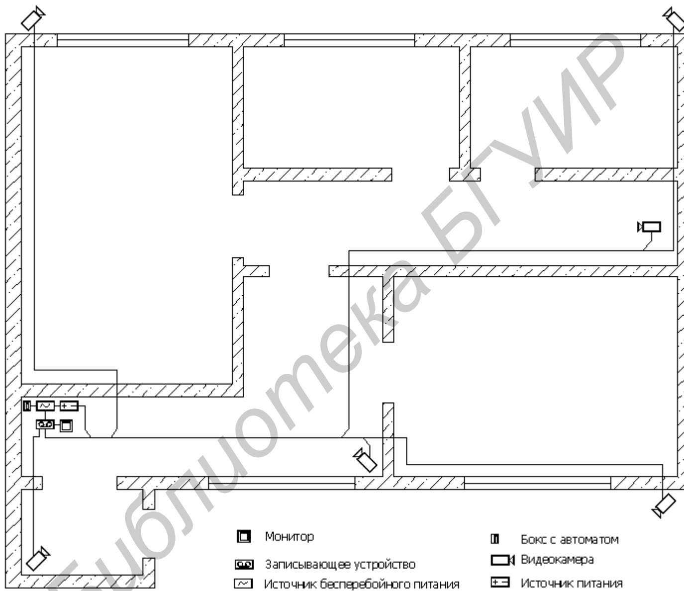
Рис. П.2. Схема размещения оборудования системы видеонаблюдения
