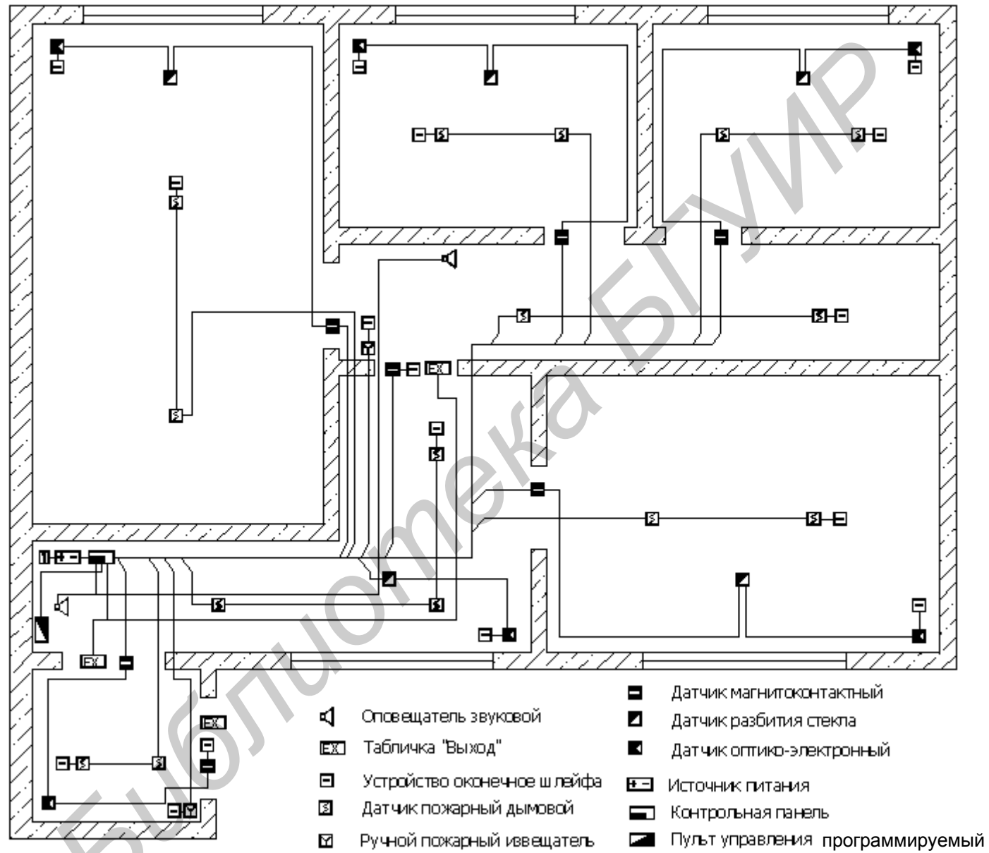
Рис. П.1. Схема размещения оборудования системы охранно-пожарной сигнализации
