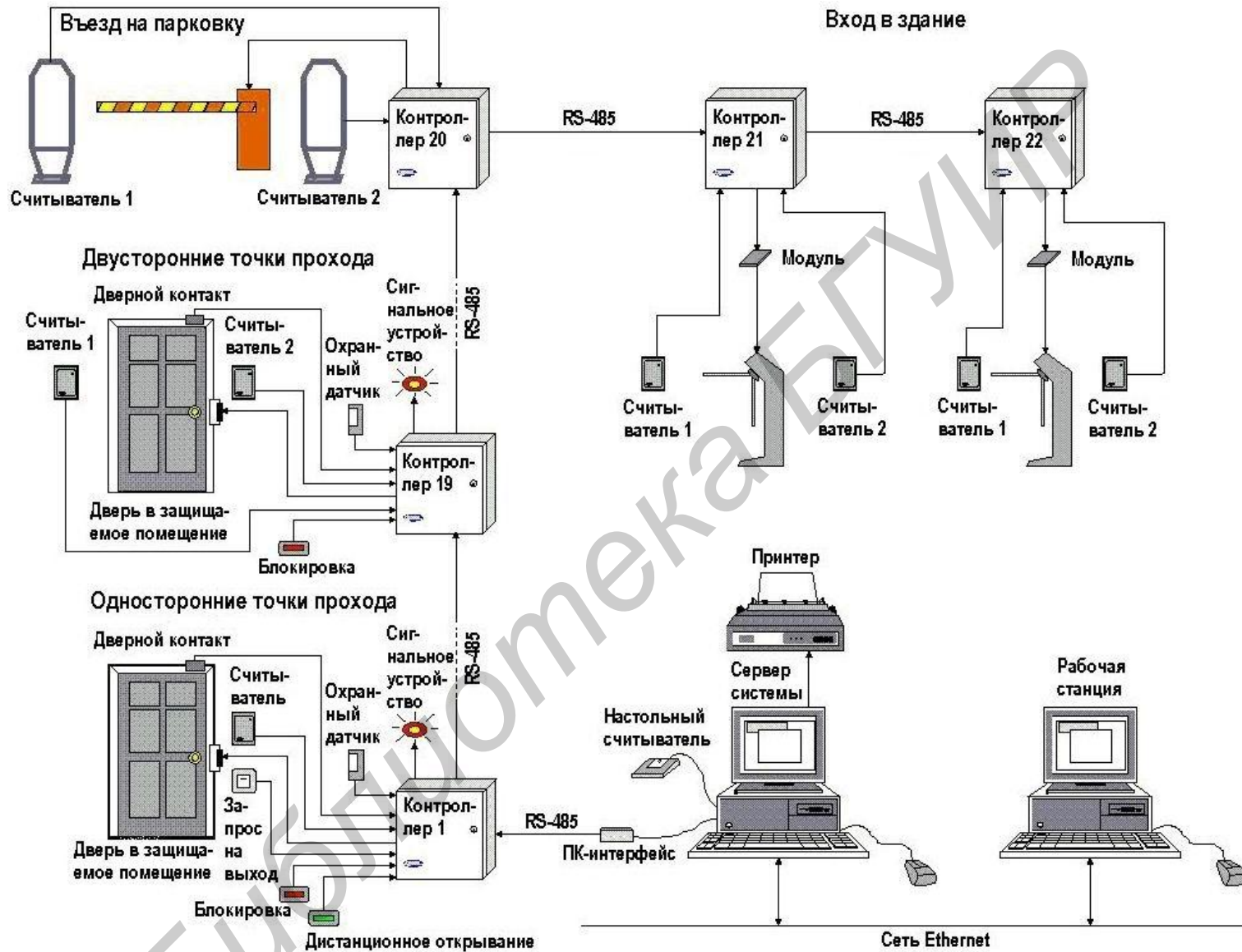
Рис. 3.3. Обобщённая структурная схема СКУД
