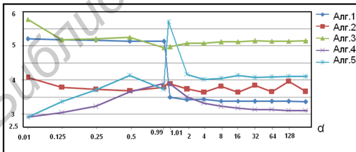
Рис. 1 – Время генерации пачки случайных чисел при различных \alpha
