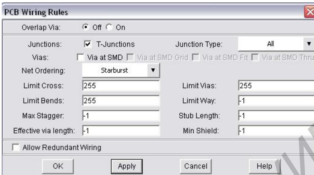
Рисунок 22 – Окно PCB Wiring Rules
