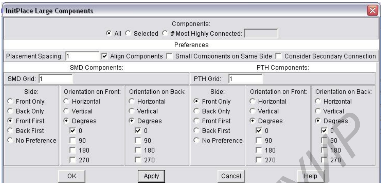
Рисунок 13 – Окно команды Autoplace/InitPlace Large Components
