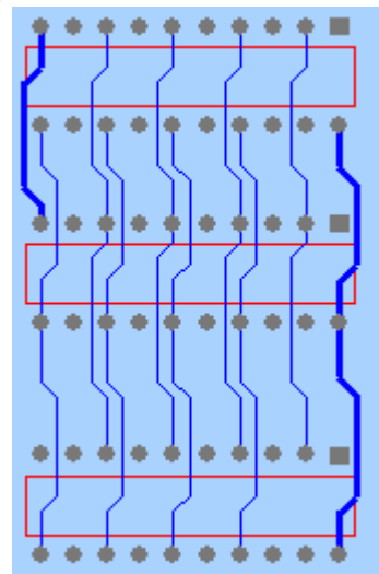
Рисунок 25 – Результат выполнения команды Autoroute/Preroute/Bus Routing
