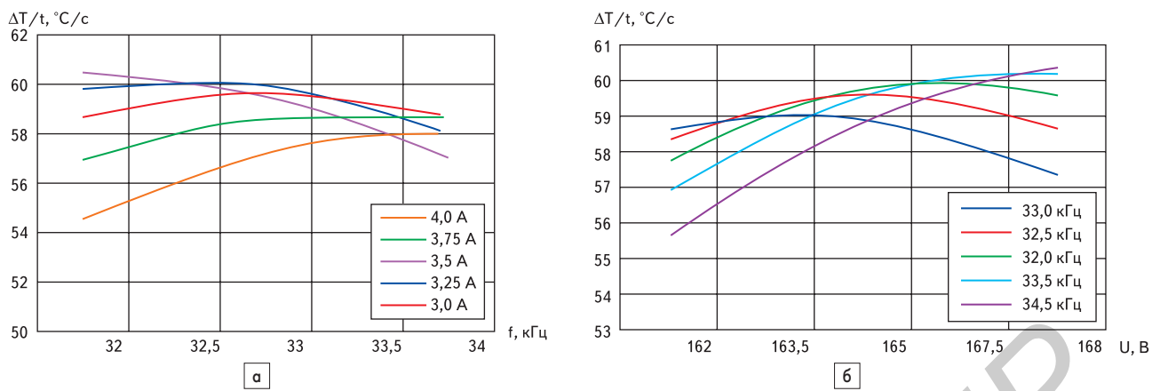
Рис. 8. Зависимости скорости нагрева при различных значениях факторов в сечениях от -1,0 до 1,0 : а — U = 165 В; б — I_n = 3,5 А: а) от частоты; б) от напряжения
