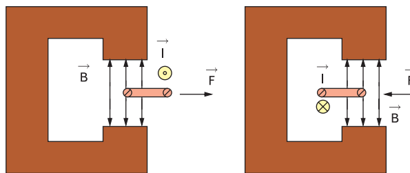
Рис. 2. Схема взаимодействия проводника с током в ЭМ поле
