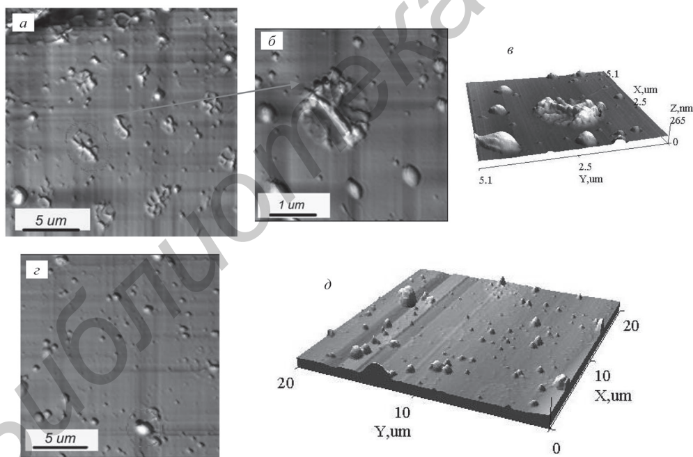
Рис. 4. 2D (а, б, с) и 3D (д, е) АСМ-изображения топографии поверхности пленки Al – 1,5 ат.% Fe, нанесенной на стекло методом ОПАСИ при отсутствии ускоряющего напряжения за 6 ч (а, б, д) и 9 ч (с, е) соответственно
