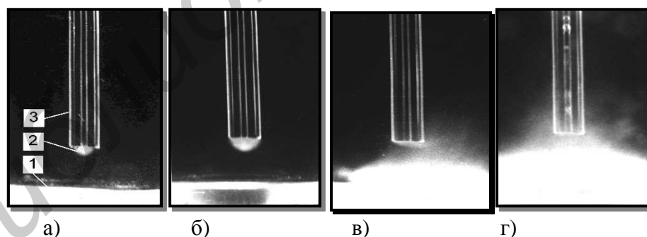
1 -- излучатель; 2 -- кавитационное облачко; 3 -- капилляр; 1 -- излучатель; 2 -- кавитационное облачко; 3 -- капилляр; А, мкм = 1(а); 2.5 (б); 6 (в); 10 (г)
