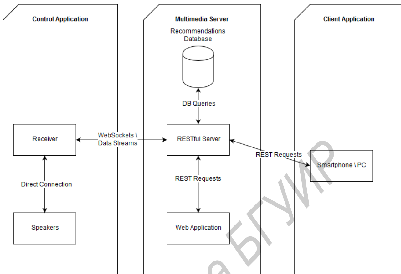
Рисунок 2 - Архитектура системы IoT-решения.
