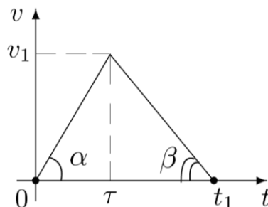
Рис. 2. График скорости изображающей точки
