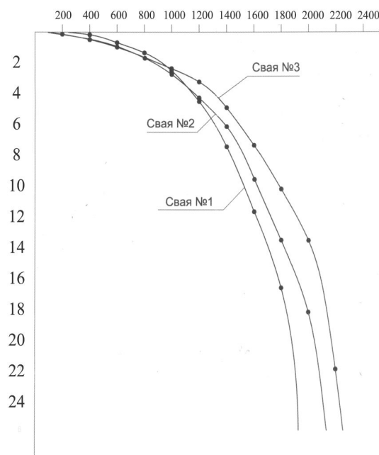
Рис. 2. Осадки РИТ-сваи от вдавливающей нагрузки
