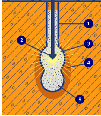
Рис. 1. Схема формирования РИТ-сваи: 1 – скважина до обработки; 2 – электродная система; 3 – зона цементации грунта; 4 – зона уплотнения грунта; 5 – камуфлетное уширение в основании РИТ-сваи
