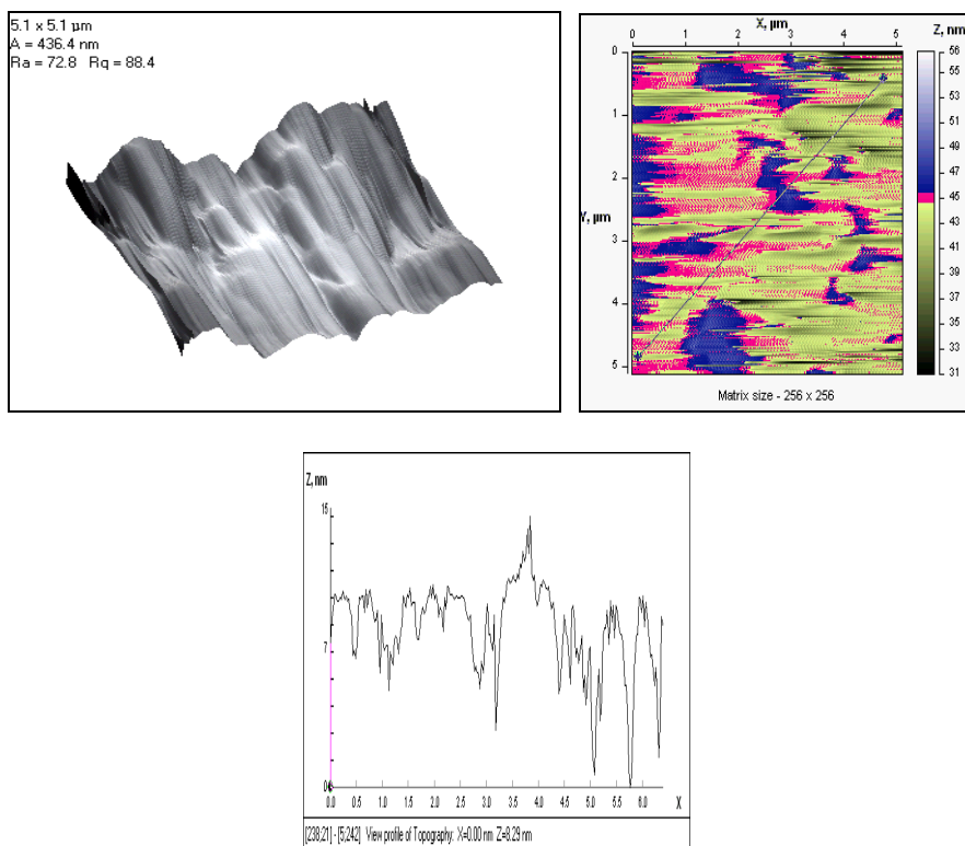
Рис. 3. АСМ-изображения: a, б ) поверхности висмутовой пленки толщиной 400 нм, напыленной при p_{O_2}=10 Па и температуре подложки 300 К; в ) профиль поверхности вдоль линии на АСМ-изображении
