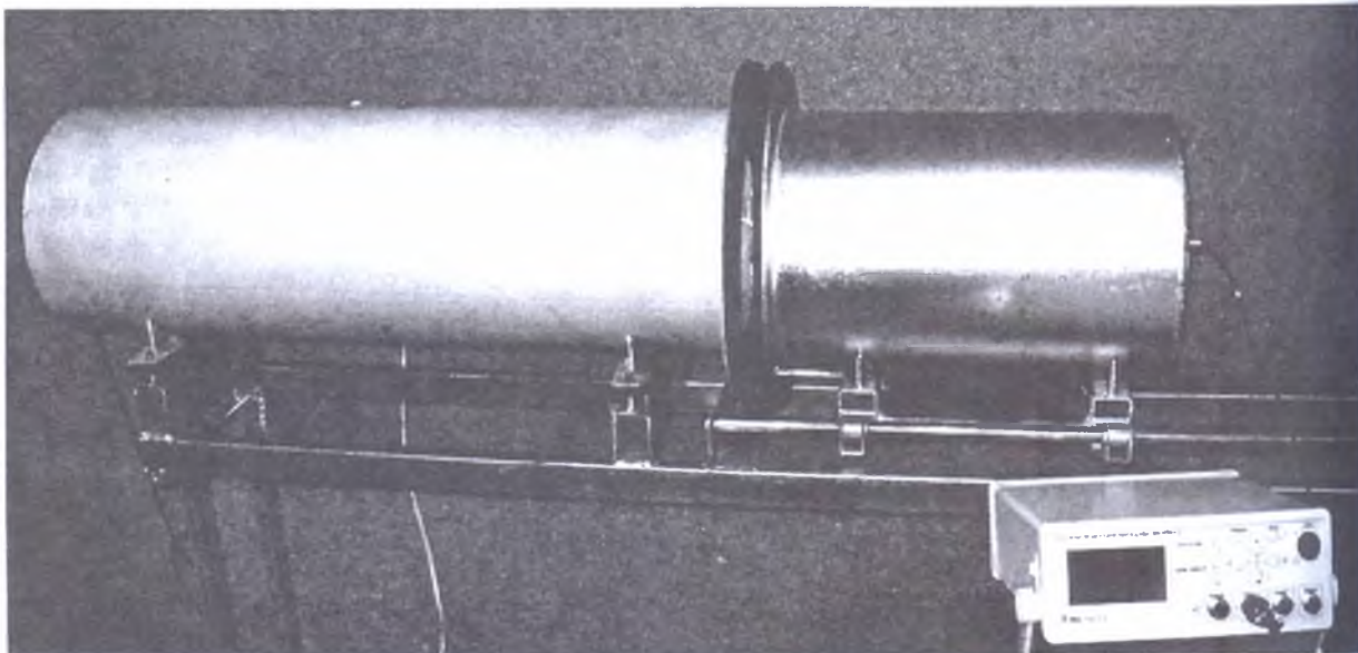
Рис. 1. Внешний вид экспериментальной установки
