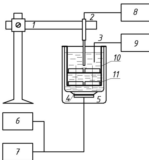
Рис. 1. Схема измерений активности кавитации: 1 – штатив, 2 – датчик, 3 – температурный датчик, 4 – пьезоэлектрический излучатель, 5 – УЗ ванна, 6 – частотомер, 7 – УЗ генератор, 8 – кавитометр, 9 – электронный термометр, 10 – проволочный держатель, 11 – образцы
