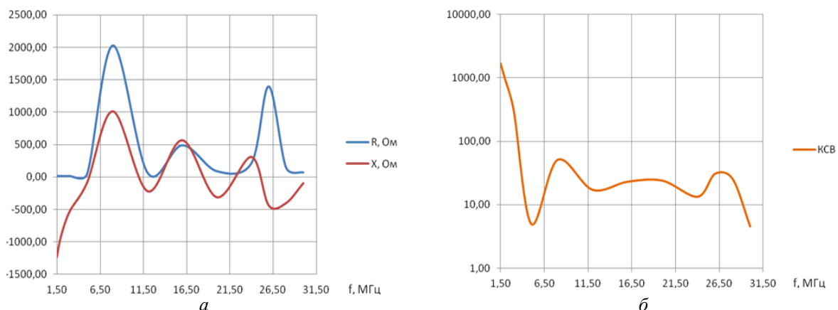
Рис. 2. Зависимость активного и реактивного сопротивления (а) и КСВ (б) антенны типа наклонный луч от частоты
