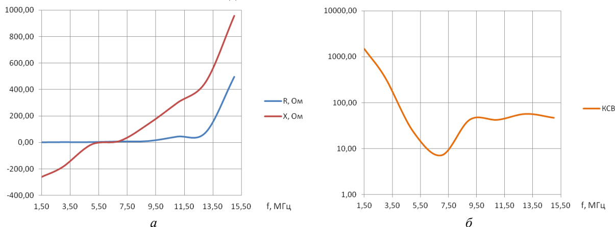
Рис. 7. Зависимость активного и реактивного сопротивления (а) и КСВ (б) дипольной ШАЗИ-2 от частоты
