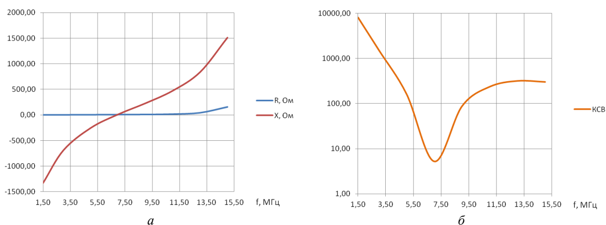
Рис. 6. Зависимость активного и реактивного сопротивления (а) и КСВ (б) дипольной АЗИ от частоты
