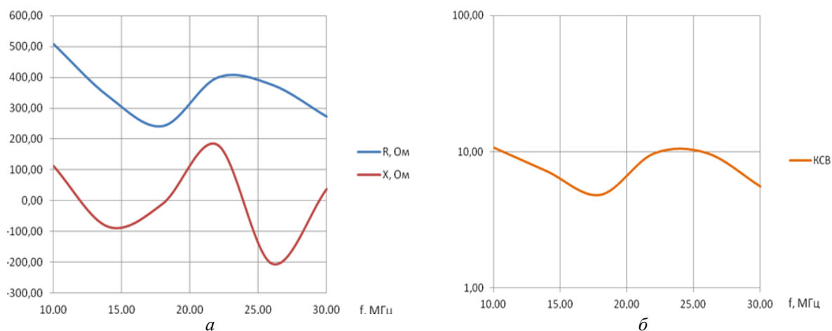
Рис. 5. Зависимость активного и реактивного сопротивления (а) и КСВ (б) антенны V2×46 от частоты
