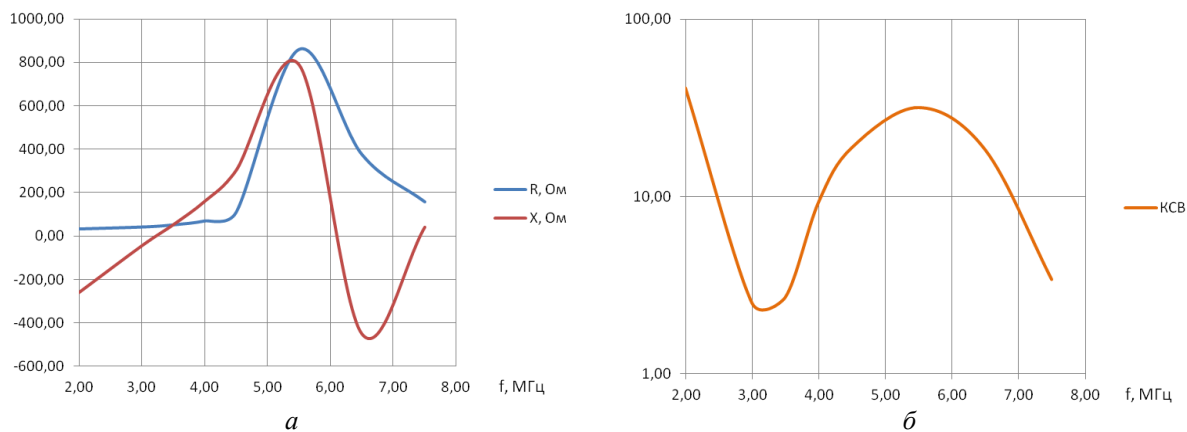
Рис. 4. Зависимость активного и реактивного сопротивления (а) и КСВ (б) антенны Т2×11 от частоты
