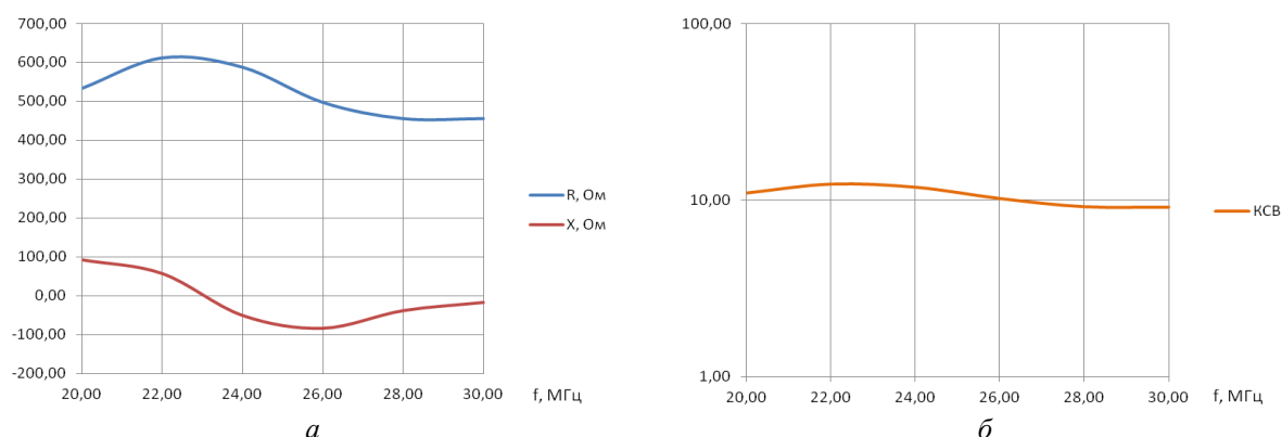
Рис. 9. Зависимость активного и реактивного сопротивления (а) и КСВ (б) антенны \lambda -15/60 от частоты
