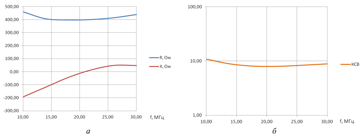
Рис. 8. Зависимость активного и реактивного сопротивления (а) и КСВ (б) антенны ОБ-40/1 от частоты
