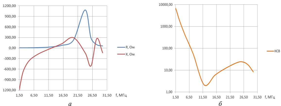
Рис. 1. Зависимость активного и реактивного сопротивления (а) и КСВ (б) антенны АШ-4 от частоты
