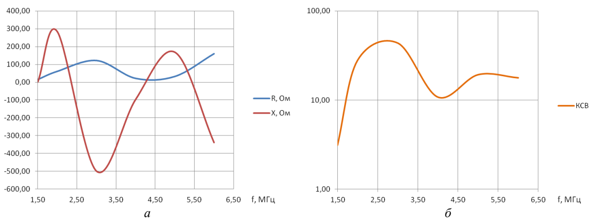
Рис. 3. Зависимость активного и реактивного сопротивления (а) и КСВ (б) антенны Д2×40 от частоты
