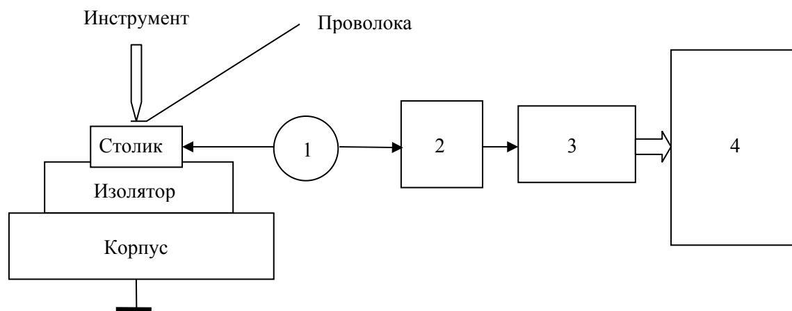
Рис. 3. Устройство контроля обрыва перемычки установки ЭМ-4371
