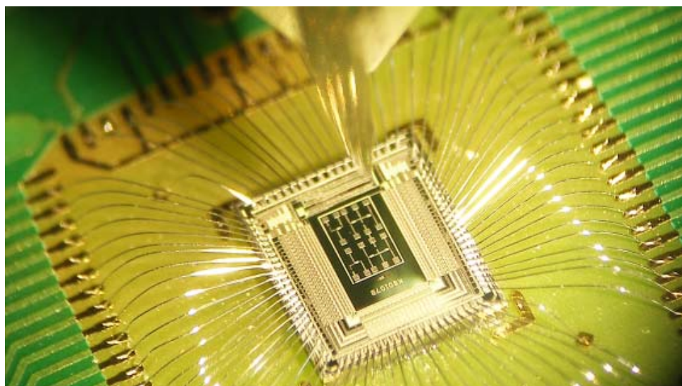
Рис. 1. Проволочный монтаж в технологии «кристалл на плате» (COB)
