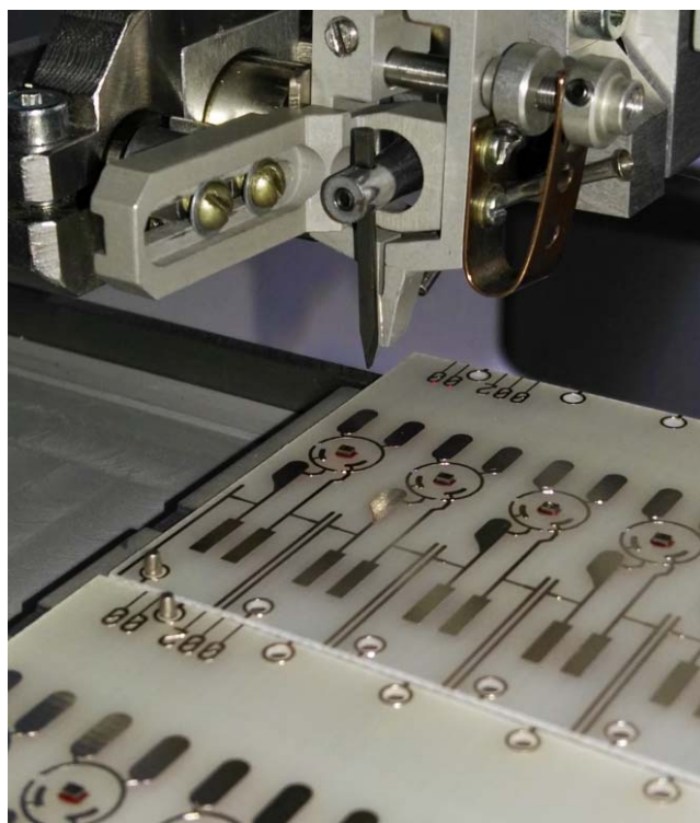
Рис. 2. Проволочный монтаж модулей корректоров на установке ЭМ-4371
