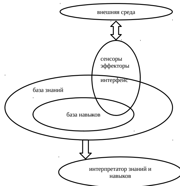
Рис. 1 – Архитектура ostis-системы
