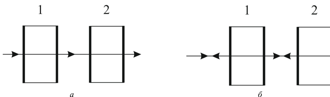
Рис. 3. Схемы преобразования ИК излучения при помощи двух микрорезонаторов Фабри–Перо: a – работающая на пропускание; b – работающая на отражение зондирующего излучения
