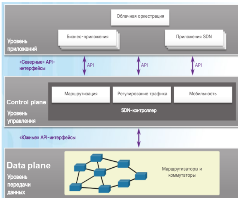
Рисунок 3 – Трехуровневая модель архитектуры SND
