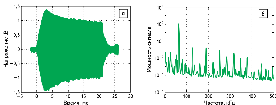
Рис. 4. Форма сигнала хорошей сварки (а) и частотный спектр мощности (б)
