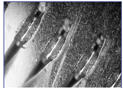
Рис. 13. Внешний вид сварных соединений алюминиевой проволокой диаметром 27 мкм
