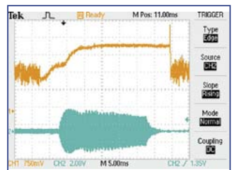
Рис. 14. Осциллограмма деформации при сварке золотой проволокой диаметром 20 мкм (верхний луч) и профиля УЗ-импульса (нижний луч)
