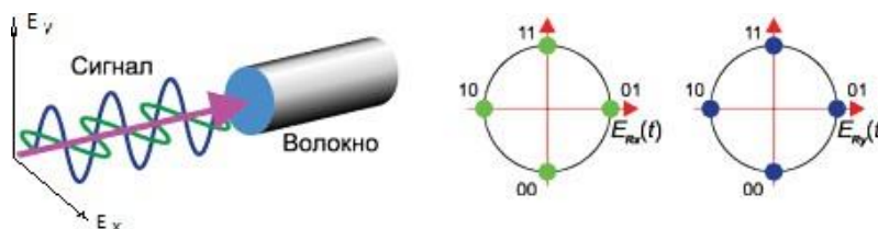
Рис. 1. Структура оптического сигнала при использовании DP-QPSK
