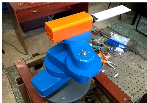
Рис. 7. Опытный образец робота-манипулятора Fig. 7. Prototype of robot-manipulator
