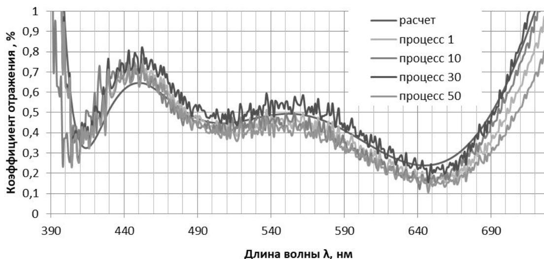
Рис. 2. Спектры отражения просветляющих покрытий без учета второй стороны стекла Fig. 2. Reflection spectra of antireflection coatings without 2 nd side of the substrate
