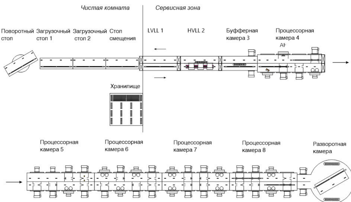
Рис. 1. Схематическое изображение линейной вакуумной установки Fig. 1. Schematic representation of a linear vacuum coater
