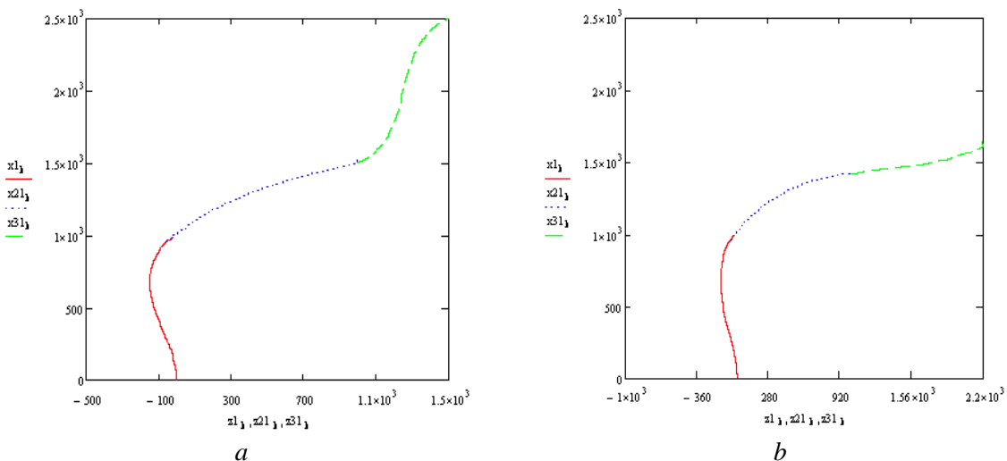
Рис. 1. Траектории полета БЛА: а – траектория, вариант 1; б – траектория, вариант 2 Fig. 1. Flight path: а – trajectory option 1; б – trajectory option 2
