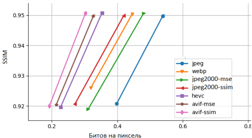
Рис. 1 - Сравнение эффективности сжатия кодеков
