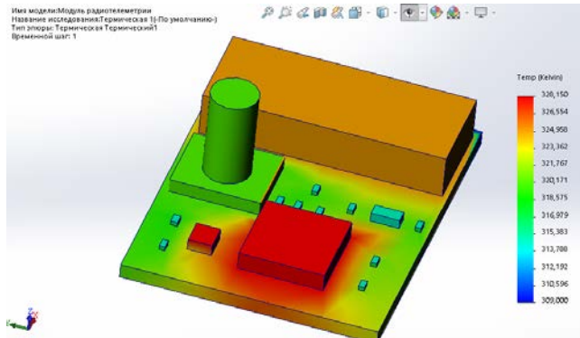
Рисунок 5 – Результаты температурного моделирования
