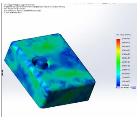
Рисунок 4 – Результаты моделирования ударных нагрузок
