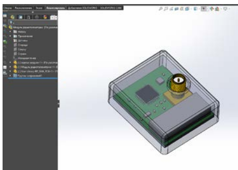
Рисунок 3 – Смоделированный в программе корпус изделия
