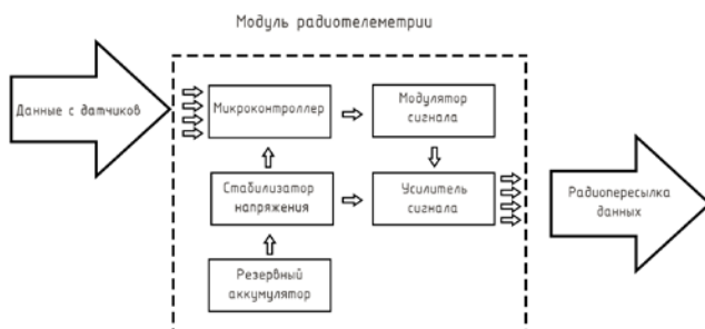
Рисунок 1 – Структурное отображение элементов модуля
