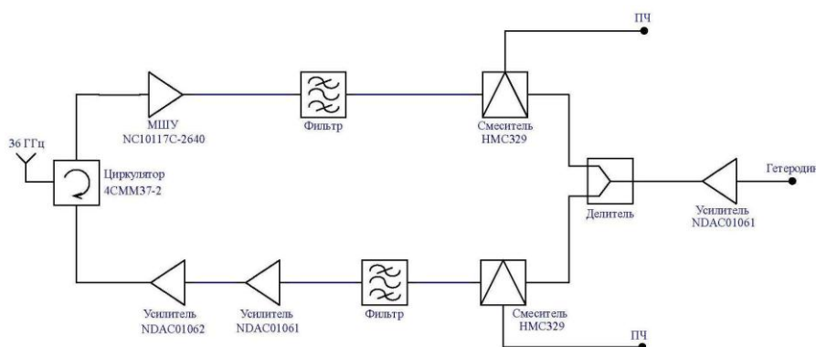
Рис. 1 – Структурная схема приемно-передающего модуля
