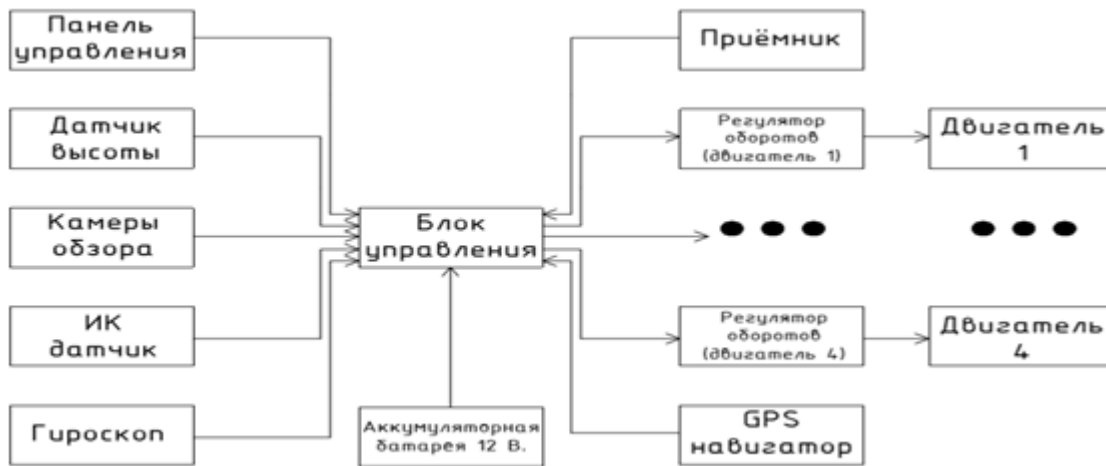
Рисунок 1– Структурная схема управления квадрокоптера
