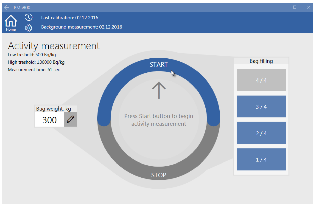
Рисунок 1 - Главный экран
