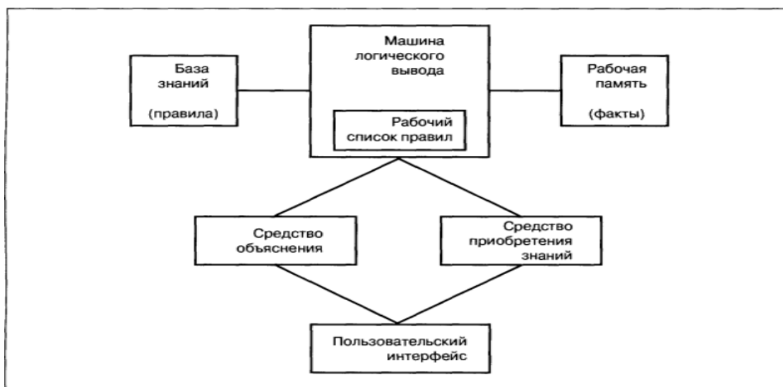
Рис.1. Структура экспертной системы, основанной на правилах[2]
