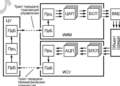
Рис. 1. Структурно-функциональная схема интеллектуальной мехатронной системы с дистанционным взаимодействием компонентов
