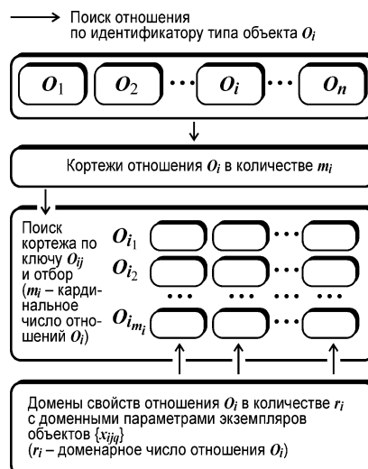
Рис. 2. Вариант построения структуры логических отношений для параметров объектов \{O_i\}
