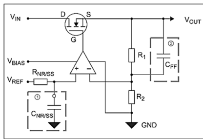
Рис. 3 – способы уменьшения шума и пульсаций выходного напряжения
