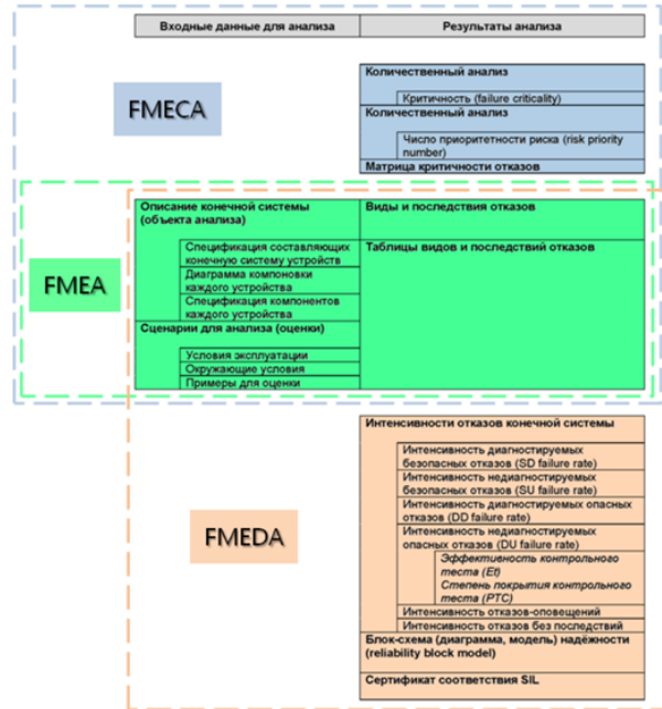
Рис. 1 – Входные данные, результаты и оценки результатов FMEA, FMESA, FMEDA
