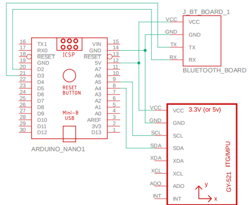
Рис. 1 – Принципиальная схема устройства
