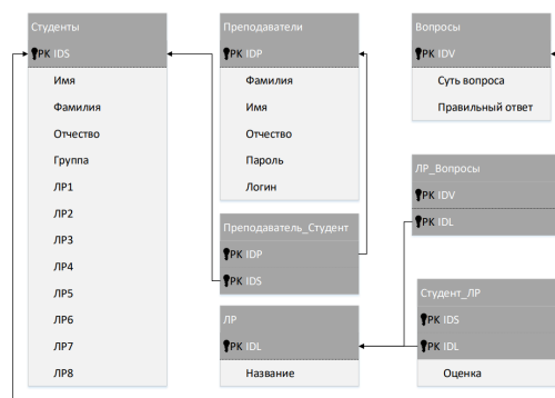
Рис. 2 – Схема баз данных
