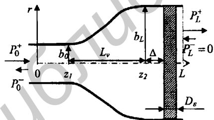
Рисунок 6 – Рупор с диэлектрической диафрагмой
