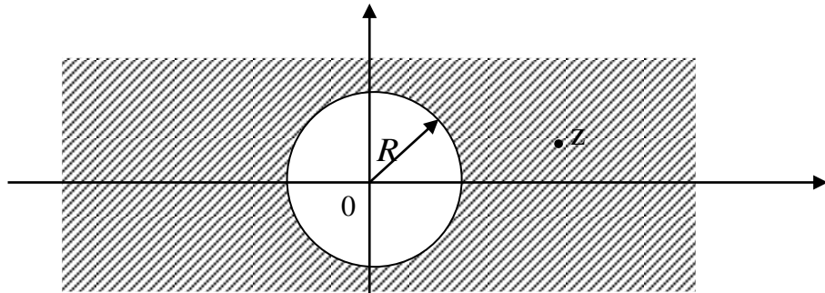
Рис. 8.2. Область сходимости ряда Лорана
