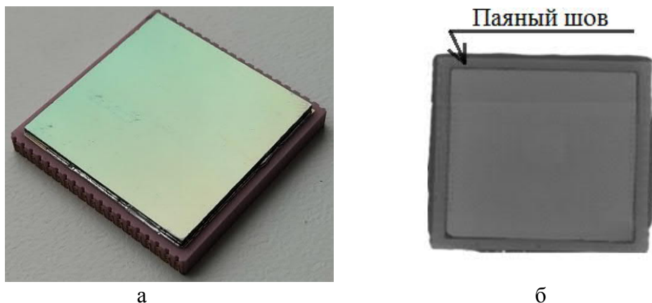
а б Рисунок 5 – Внешний загерметизированного корпуса микроболометра
