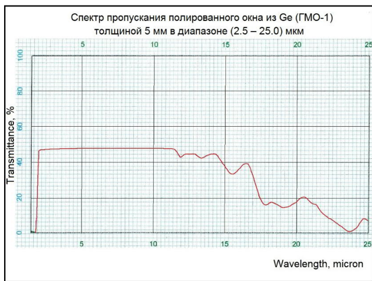
Рисунок 3 – Спектр пропускания монокристаллического германия
