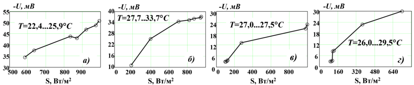
а – структура \text{Si} / \text{Ni} / \text{SiO}_2 : \text{Cu}^+ / \text{Ni} , б – структура \text{Si} / \text{Ni} / \text{SiO}_2 : \text{Cu}^+ : \text{Zn}^+ / \text{Ni} , в – структура \text{Si} / \text{Ni} / \text{SiO}_2 : \text{NiO} / \text{Ni} , з – структура \text{Si} / \text{Ni} / \text{SiO}_2 : \text{CuO} / \text{Ni}
