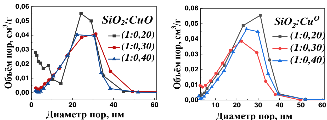
Рисунок 1 – Изотермы распределения размеров пор для изучаемых образцов микророшков
