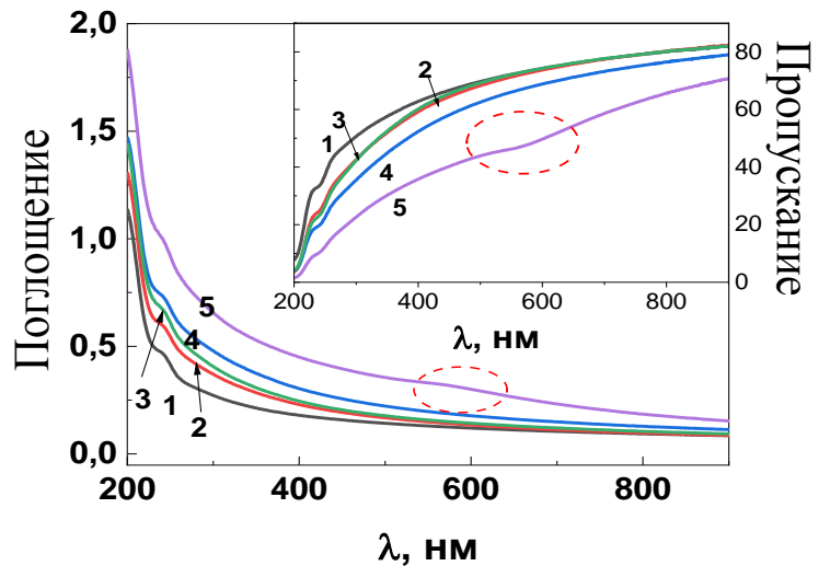
1 – подложка, 2 – \text{SiO}_2 , 3 – (1 : 0,20), 4 – (1 : 0,30), 5 – (1 : 0,40)
