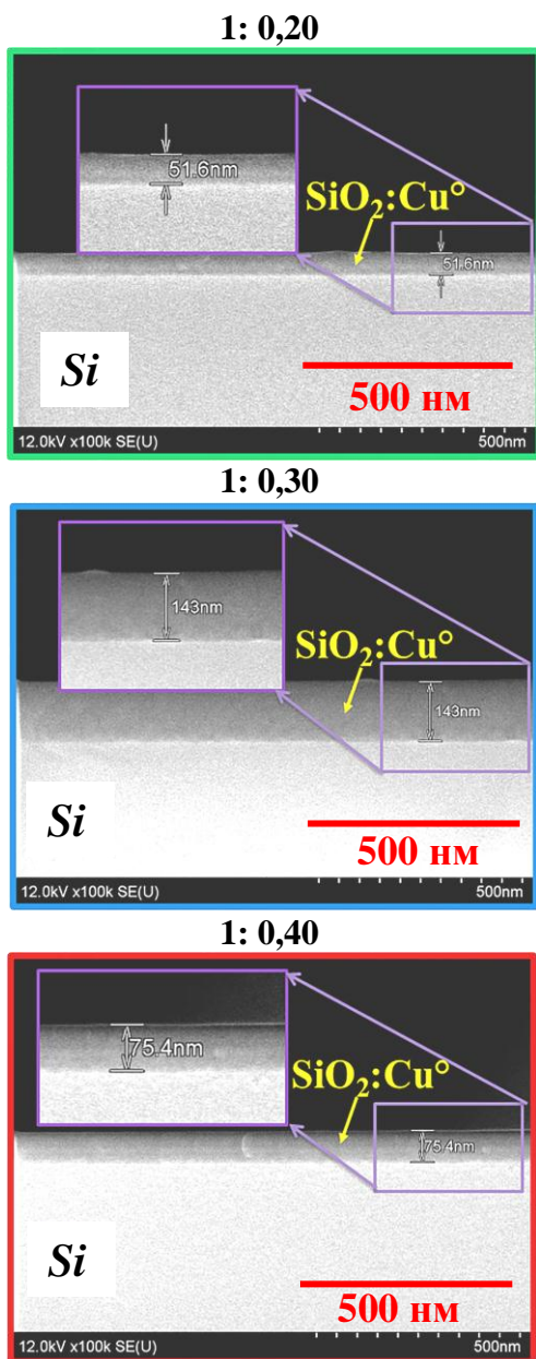
Рисунок 7 – СЭМ-изображение скола пленки, \text{SiO}_2 : \text{Cu}^\circ
