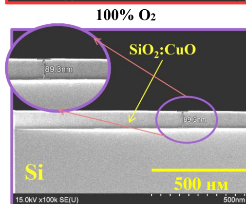
Рисунок 6 – СЭМ-изображение поверхности скола тонкой пленки, нанесенной методом ионно-лучевого распыления мишени состава SiO 2 :CuO на подложке из полированного кремния при различном составе рабочего газа
