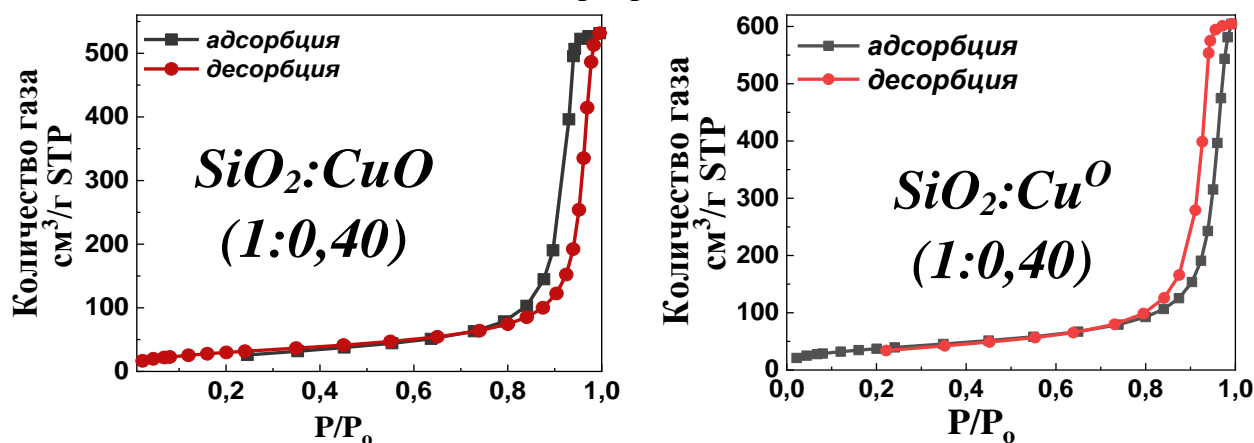
Рисунок 2 – Изотермы низкотемпературной адсорбции-десорбции азота изучаемых образцов микророшков
