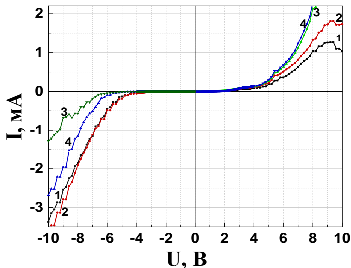
1– \text{SiO}_2 , 2– (1 : 0,20), 3– (1 : 0,30), 4 – (1 : 0,40) Рисунок 8 – Вольт-амперные характеристики для \text{SiO}_2 , \text{SiO}_2 : \text{Cu}^\circ пленок
