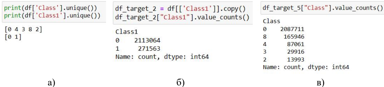
Рисунок 5. Описание целевых признаков: а) уникальные значения целевых признаков, б) и в) число объектов с уникальными значениями для целевых признаков
