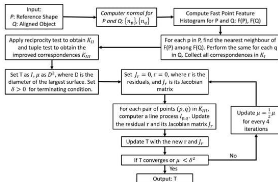
Рисунок 4. Рабочий процесс FGR .
