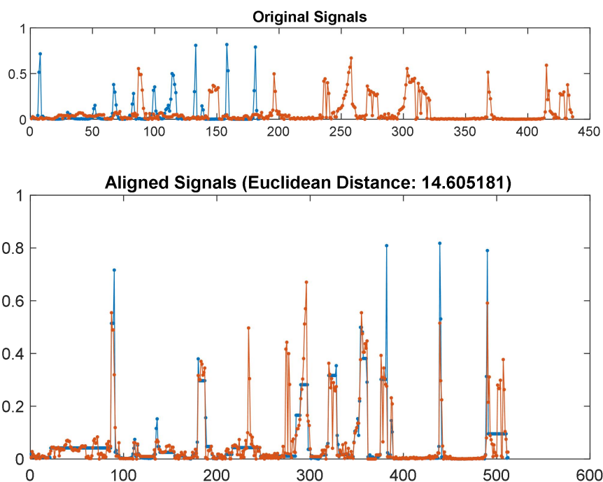
Рисунок 4. Совмещение двух параметрически заданных функций с помощью преобразования dtw
