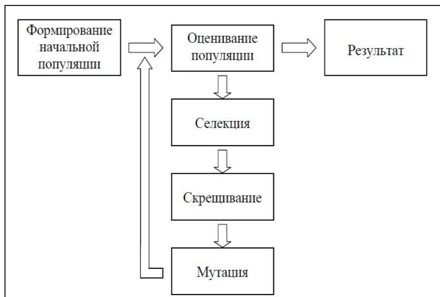
Рисунок 3. Генетический алгоритм
