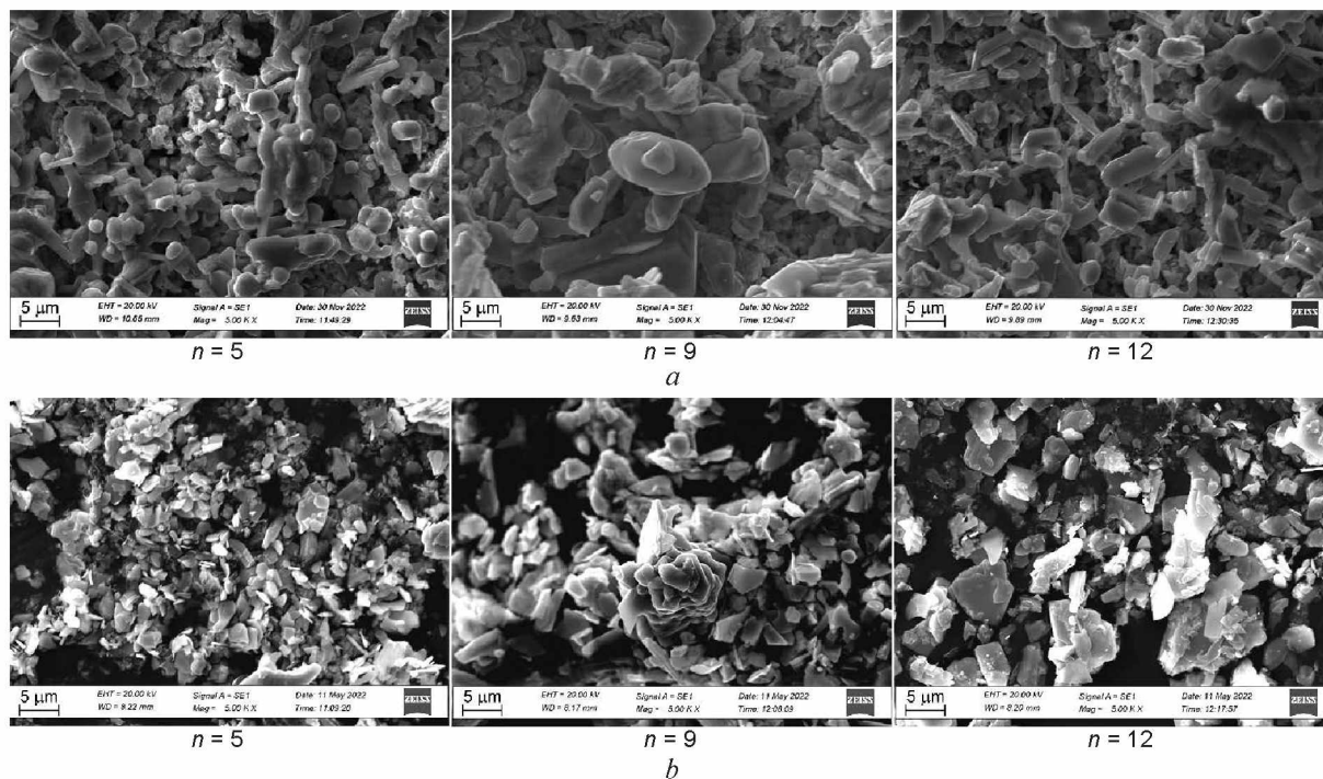
Рис. 3. Микрофотографии поверхности образцов сегнетоэлектрик–высокотемпературный сверхпроводник: a – из синтезированного высокотемпературного сверхпроводникового материала; b – из прекурсоров Fig. 3. Microphotographs of the surface of ferroelectric samples – high-temperature superconductor: a – from synthesized high-temperature superconducting material; b – from precursors
