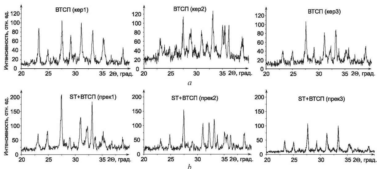
Рис. 2. Дифрактограммы образцов: a - \text{ВТСП} ; b - \text{ST+ВТСП} (из прекурсоров): ВТСП – высокотемпературный сверхпроводник; ST – \text{SrTiO}_3 Fig. 2. X-ray diffraction patterns of samples: a - \text{HTSC} ; b - \text{ST+HTSC} (from precursors): HTSC – high temperature superconductor; ST – \text{SrTiO}_3
