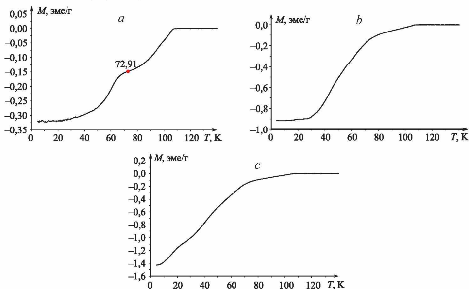
Рис. 1. Температурные зависимости намагниченности сверхпроводников на основе \text{Bi}_{1,7}\text{Pb}_{0,3}\text{Sr}_2\text{Ca}_{(n-1)}\text{Cu}_n\text{O}_y для n : a - 5 ; b - 9 ; c - 12 Fig. 1. Temperature dependences of the magnetization of superconductors based on \text{Bi}_{1,7}\text{Pb}_{0,3}\text{Sr}_2\text{Ca}_{(n-1)}\text{Cu}_n\text{O}_y for n : a - 5 ; b - 9 ; c - 12
