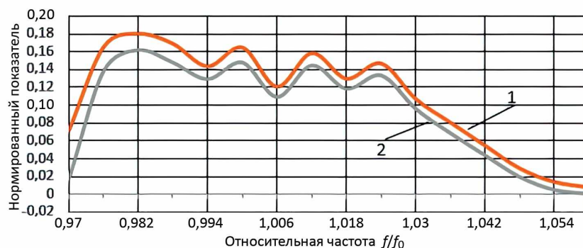
Рис. 6. Частотная характеристика gyro-ЛБВ-умножителя частоты: 1 – КПД-Е; 2 – КПД-В Fig. 6. Frequency response of gyro-TWT frequency multiplier: 1 – efficiency-E; 2 – efficiency-V
