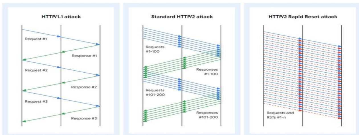
Рисунок 1 – Механизмы реализации DoS и DDoS кибератак с использованием различных версий протокола HTTP
