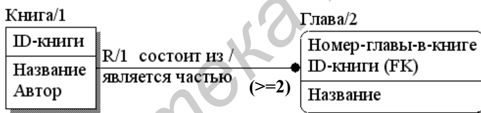
Рис. 5.28. Графическое представление в IDEF1X связи мощностью один-к-(условие)
