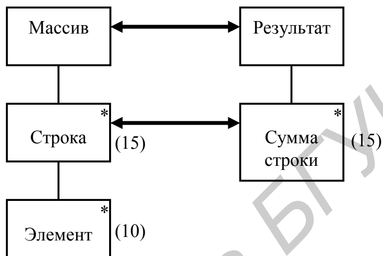
Рис. 4.43. Соответствие между структурами входных и выходных данных
