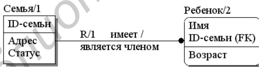
Рис. 5.24. Графическое представление в IDEF1X связи мощностью один-к-нулю-одному-или-многим
