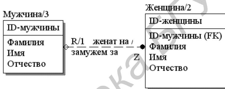
Рис. 5.33. Графическое представление в IDEF1X необязательной идентифицирующей связи мощностью ноль-или-один-к-нулю-или-одному
