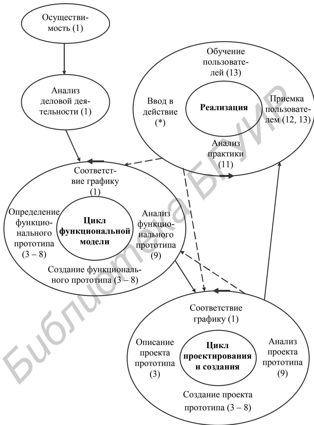
Рис. 2.11. Вариант модели быстрой разработки приложений по ГОСТ Р ИСО/МЭК ТО 15271–2002
