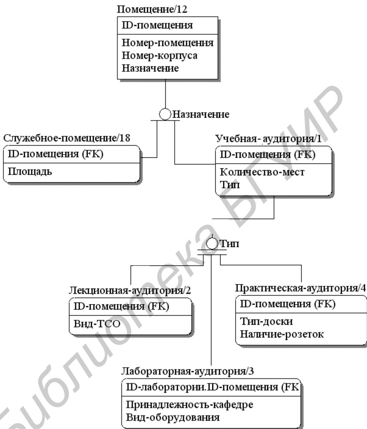
Рис. 5.45. Вложенность связей категоризации. Использование имени предка в качестве имени унаследованного идентификатора
