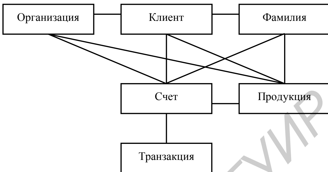
Рис. 4.38. Пример сетевой структуры данных
