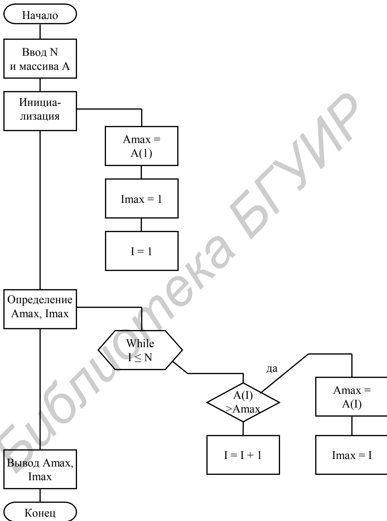
Рис. 4.13. Схема алгоритма поиска максимального элемента массива и его номера, представленная по методу Дамке
