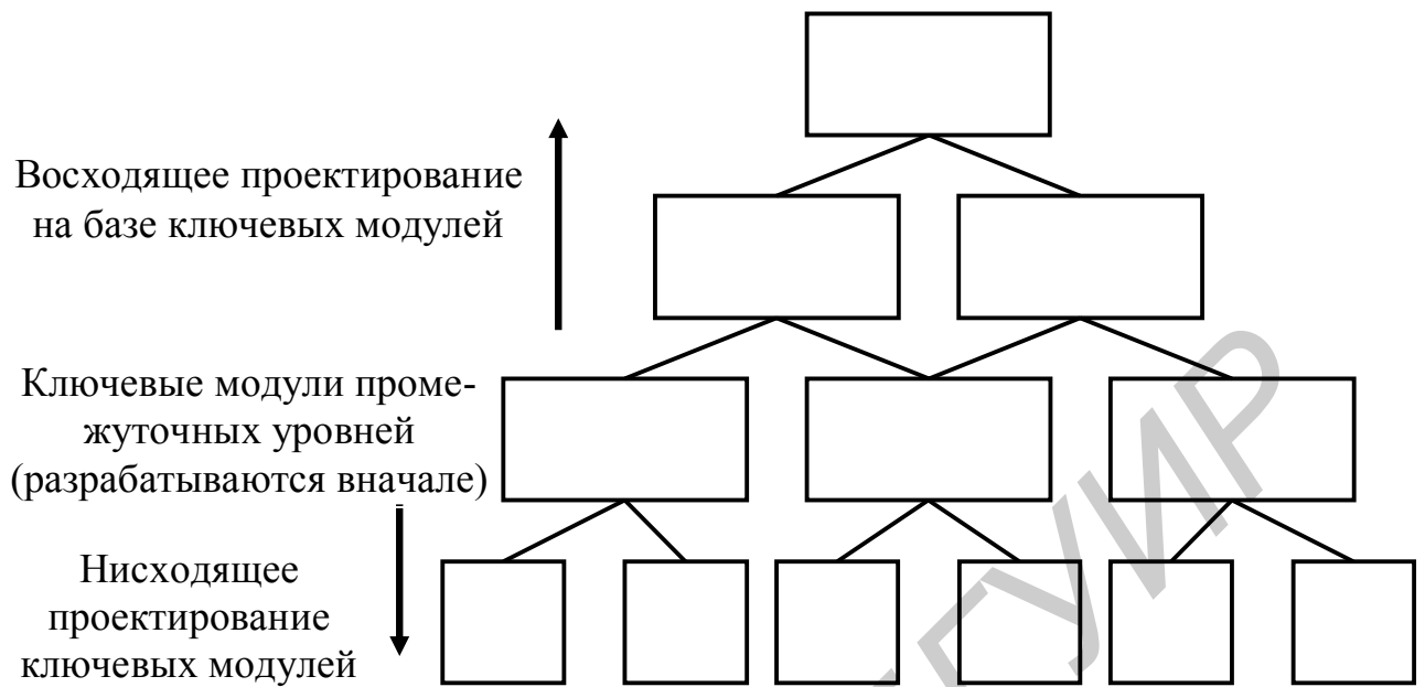
Рис. 4.27. Проектирование программы нисходящим и восходящим методами на базе ключевых модулей
