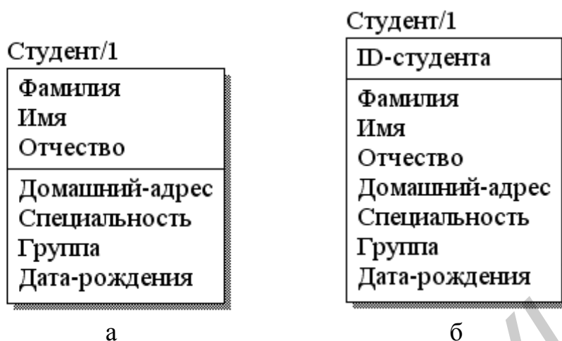
Рис. 5.19. Графическое представление сущности Студент: а – с использованием составного идентификатора; б – с использованием идентификационного номера
