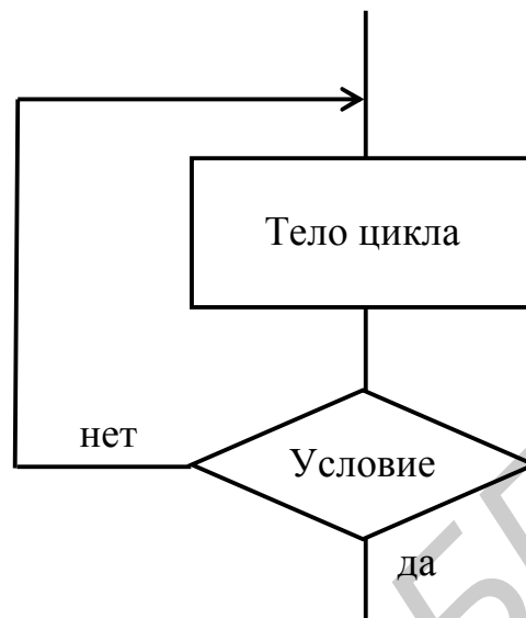
Рис. 4.5. Изображение цикла с постусловием в структурном программировании
