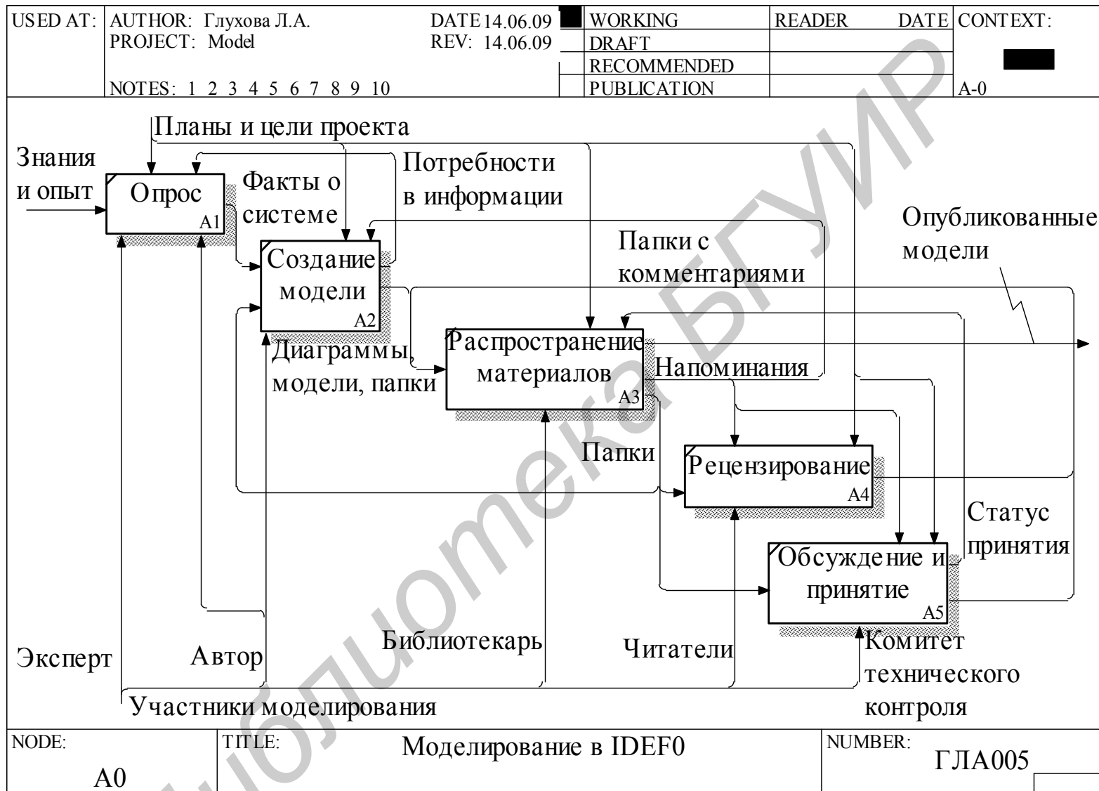
Рис. 5.11. Процесс моделирования в IDEF0
