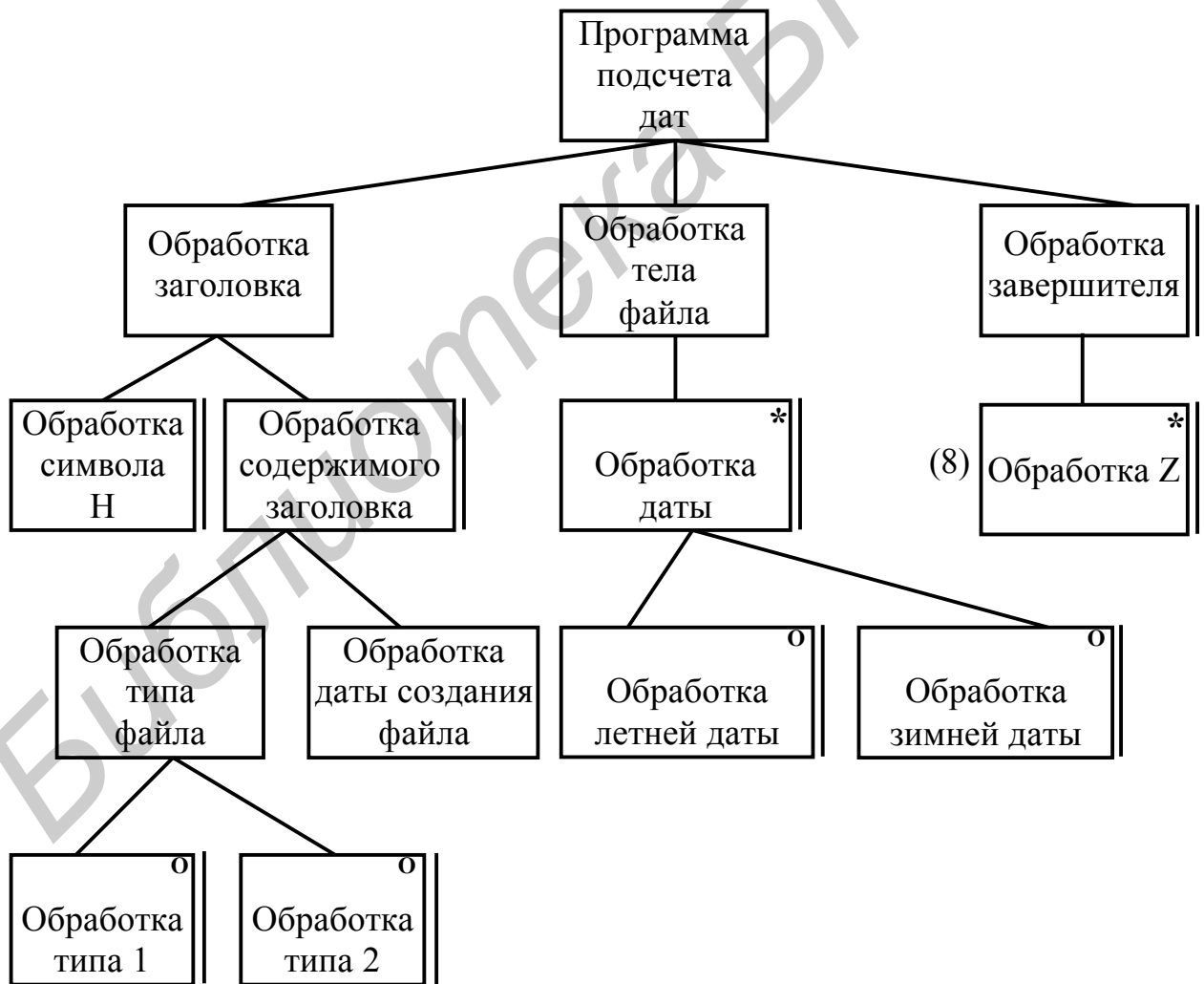
Рис. 4.53. Добавление не имеющих соответствия компонентов структуры входных данных
