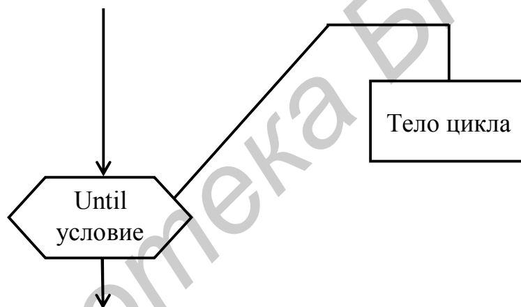
Рис. 4.10. Представление цикла с постусловием по методу Дамке
