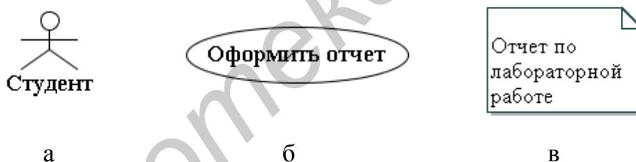
Рис. 6.1. Графическое представление основных элементов диаграммы вариантов использования:
