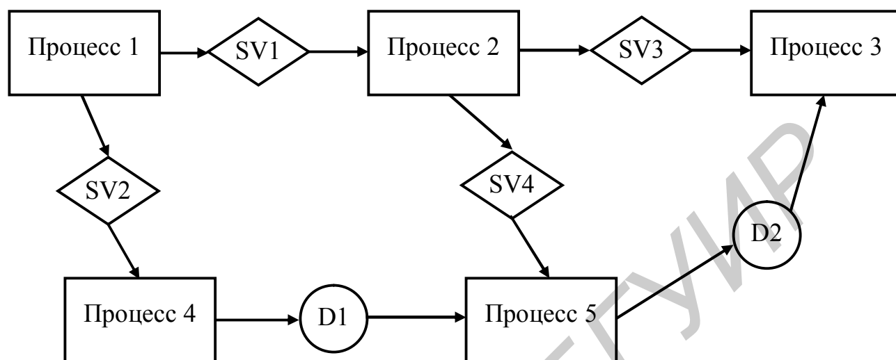
Рис. 5.50. Общий вид ND-диаграммы
