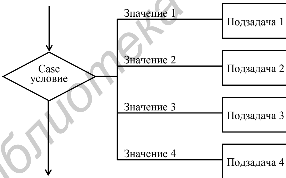
Рис. 4.12. Представление конструкции Case по методу Дамке
