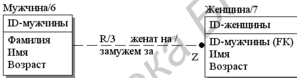
Рис. 5.31. Графическое представление в IDEF1X неидентифицирующей связи мощностью один-к-нулю-или-одному
