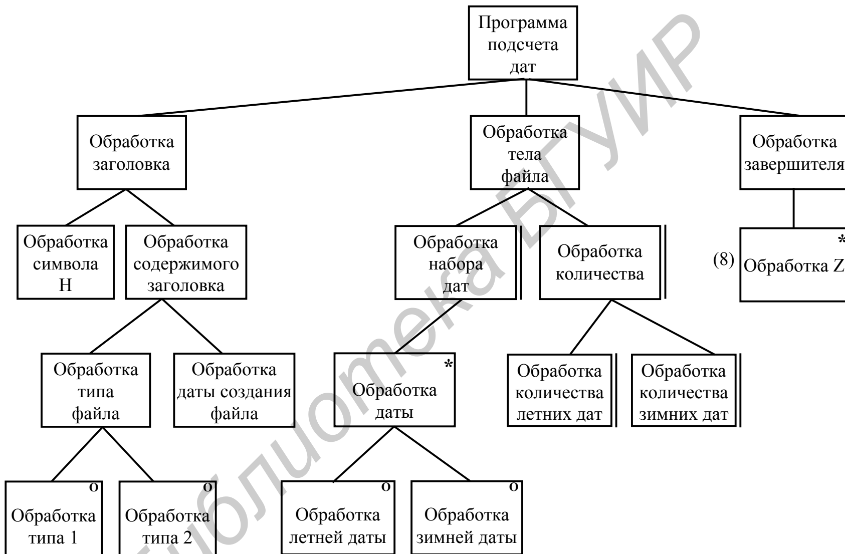
Рис. 4.54. Добавление не имеющих соответствия компонентов структуры выходных данных
