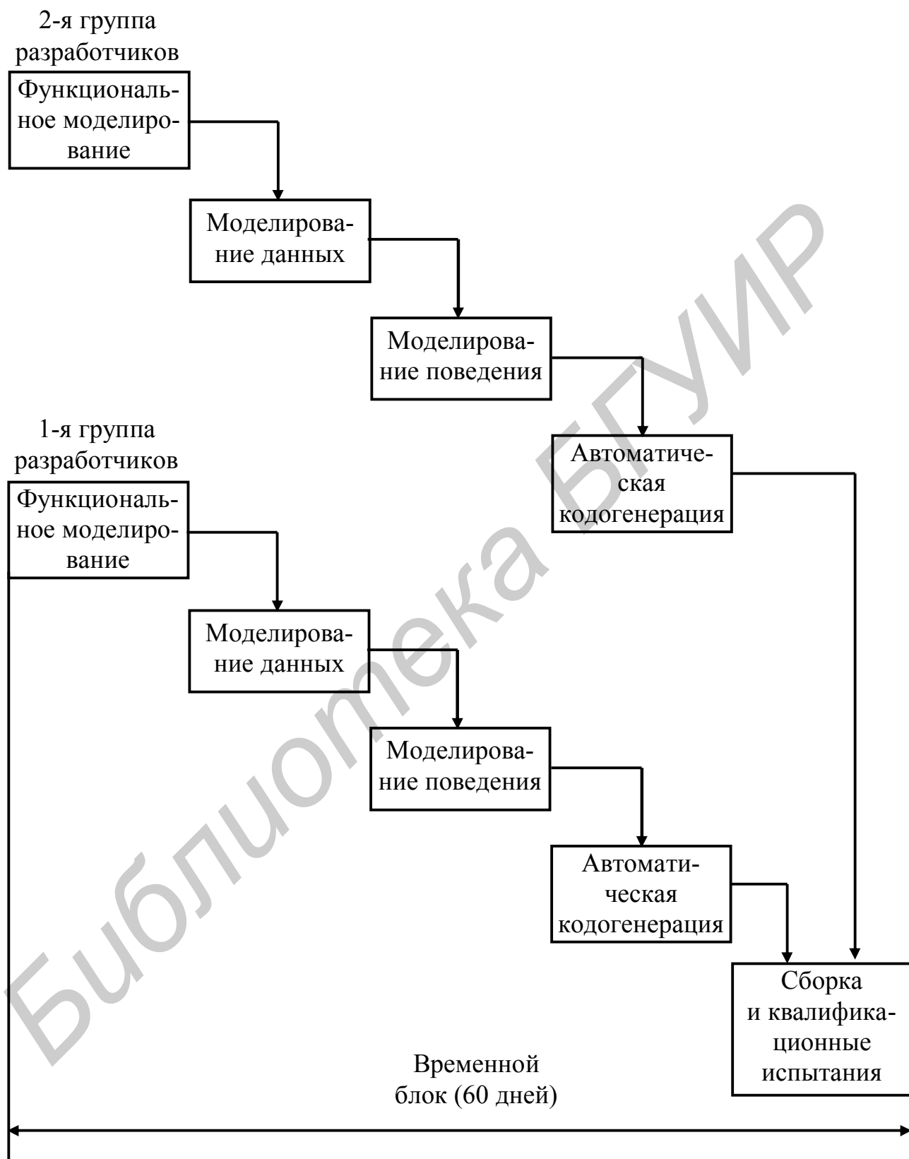
Рис. 2.10. Вариант RAD-модели, основанный на независимой работе групп разработчиков
