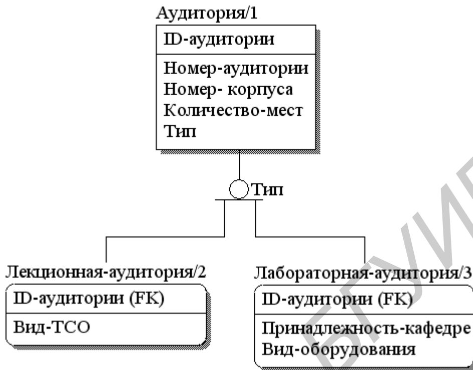
Рис. 5.44. Связь категоризации. Неполная группа категорий
