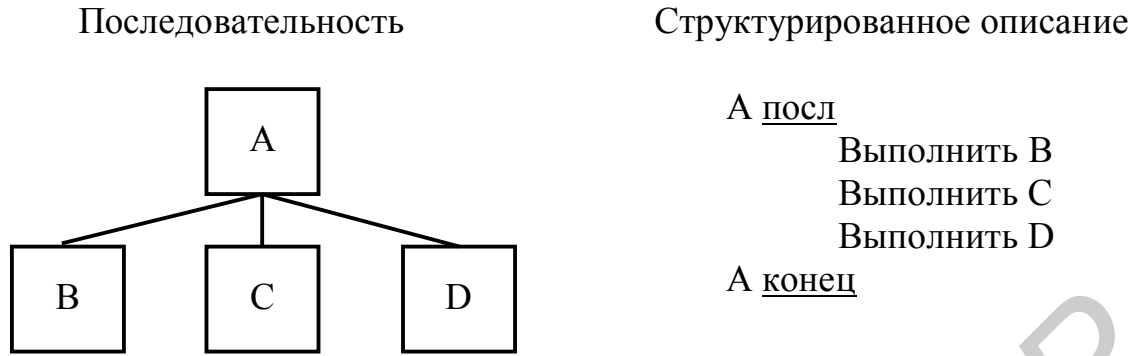
Рис. 4.56. Конструкция последовательности и ее структурированное описание
