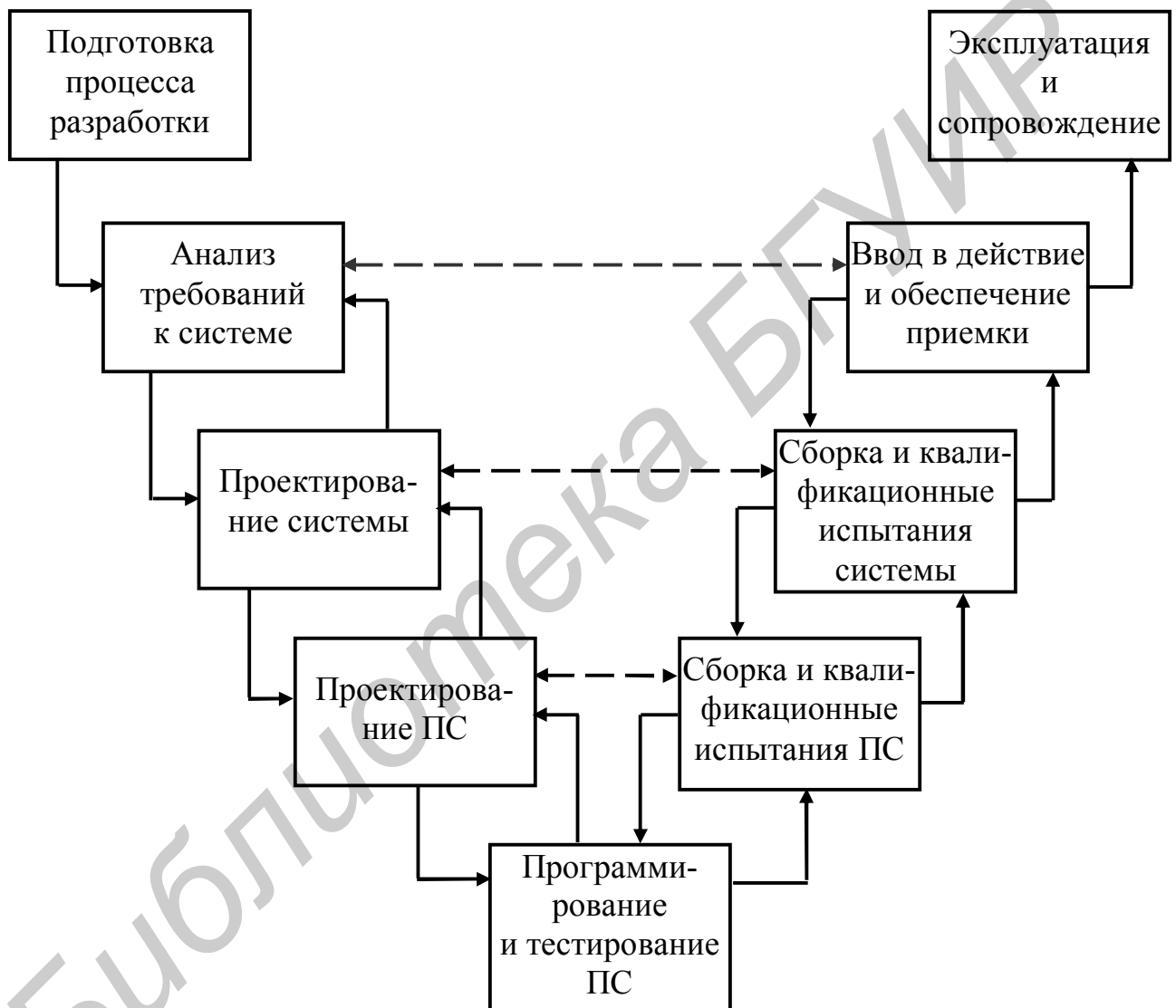
Рис. 2.7. V-образная модель жизненного цикла с организацией обратных связей между соседними этапами
