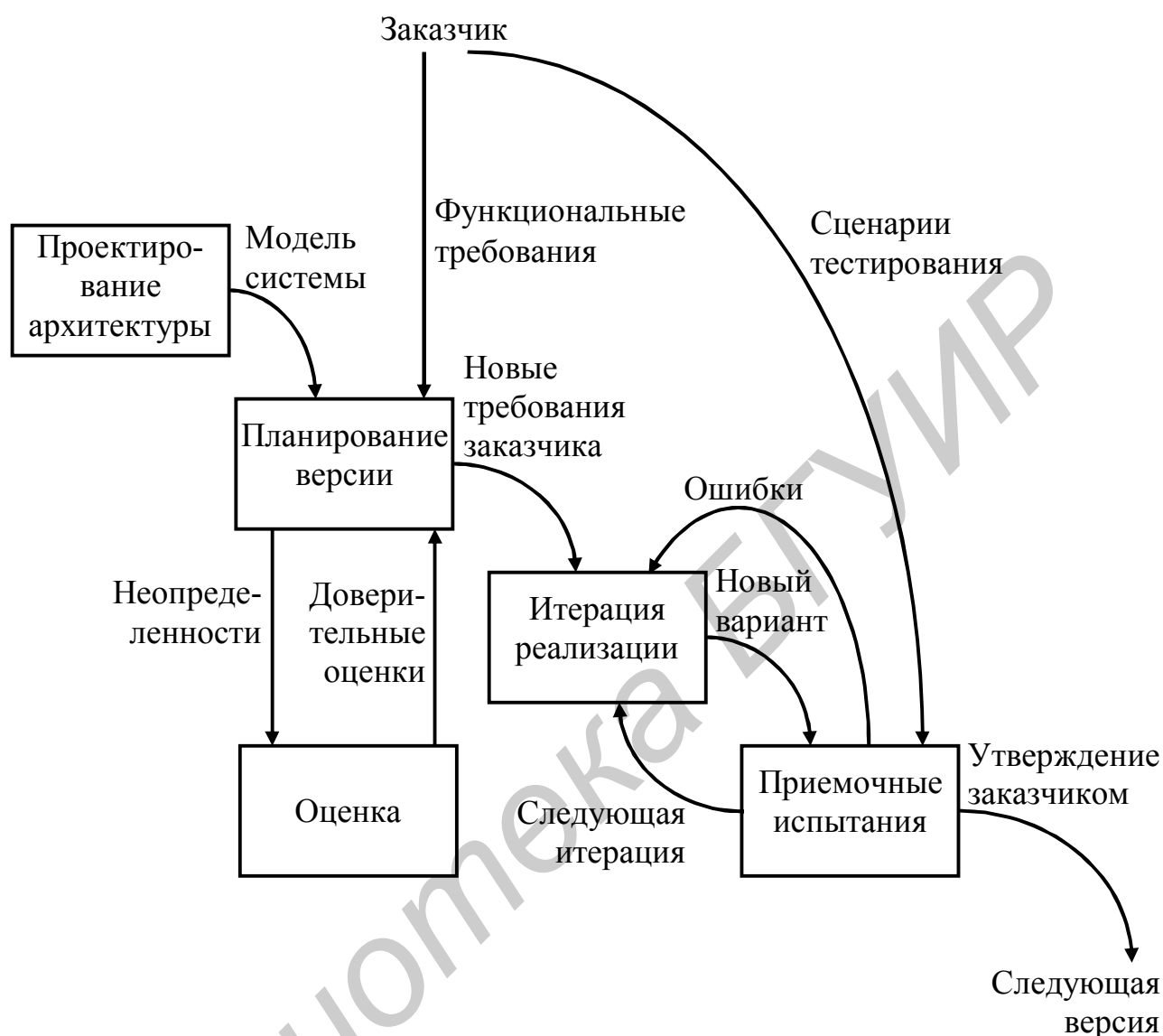
Рис. 2.14. Вариант инкрементной модели экстремального программирования
