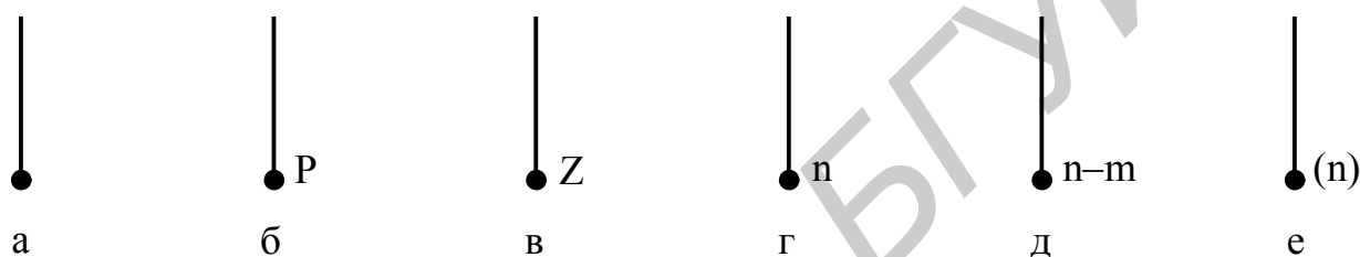
Рис. 5.23. Графическое представление различных видов дочерней мощности соединительных связей в IDEF1X:
