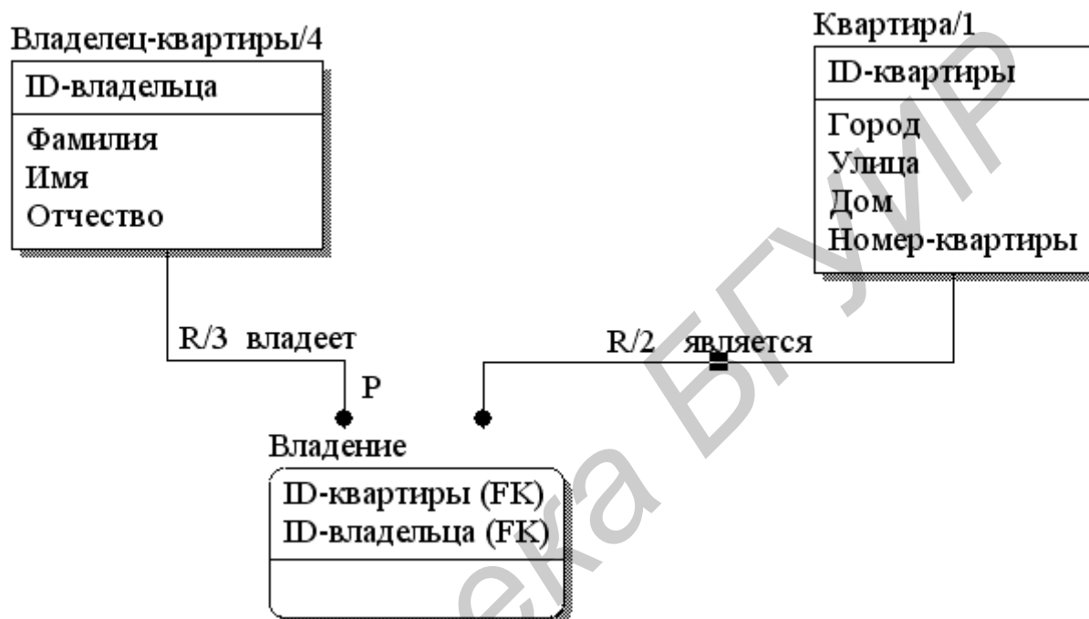
Рис. 5.35. Формализация связи многие-ко-многим посредством ассоциативной сущности
