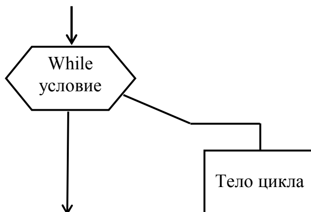
Рис. 4.9. Представление цикла с предусловием по методу Дамке
