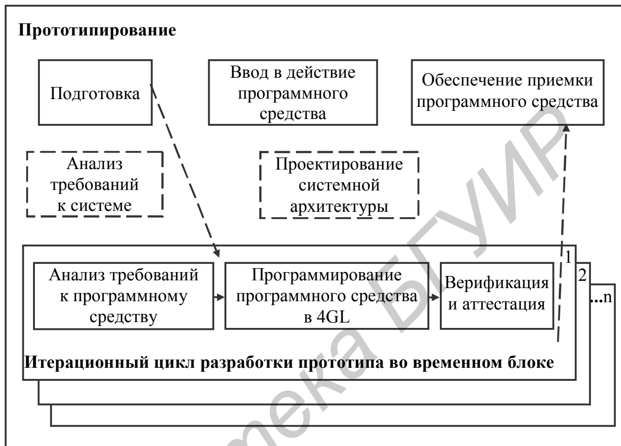
Рис. 2.17. Вариант эволюционной модели прототипирования по ГОСТ Р ИСО/МЭК ТО 15271–2002
