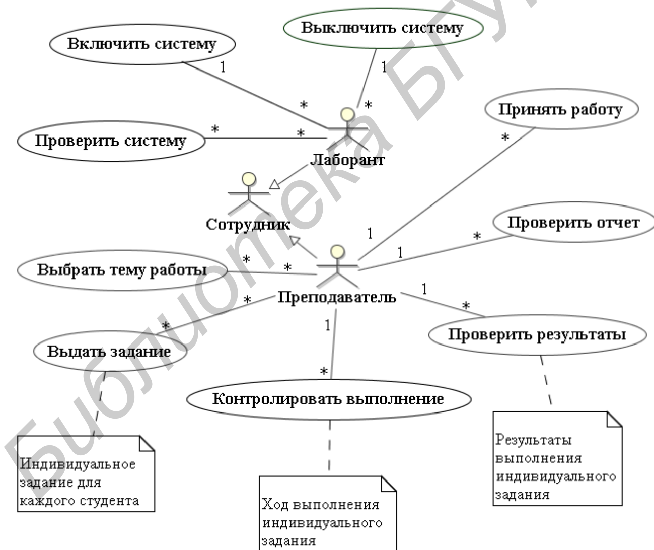
Рис. 6.2. Диаграмма вариантов использования системы автоматизации выполнения лабораторных работ для актеров «Преподаватель» и «Лаборант»
