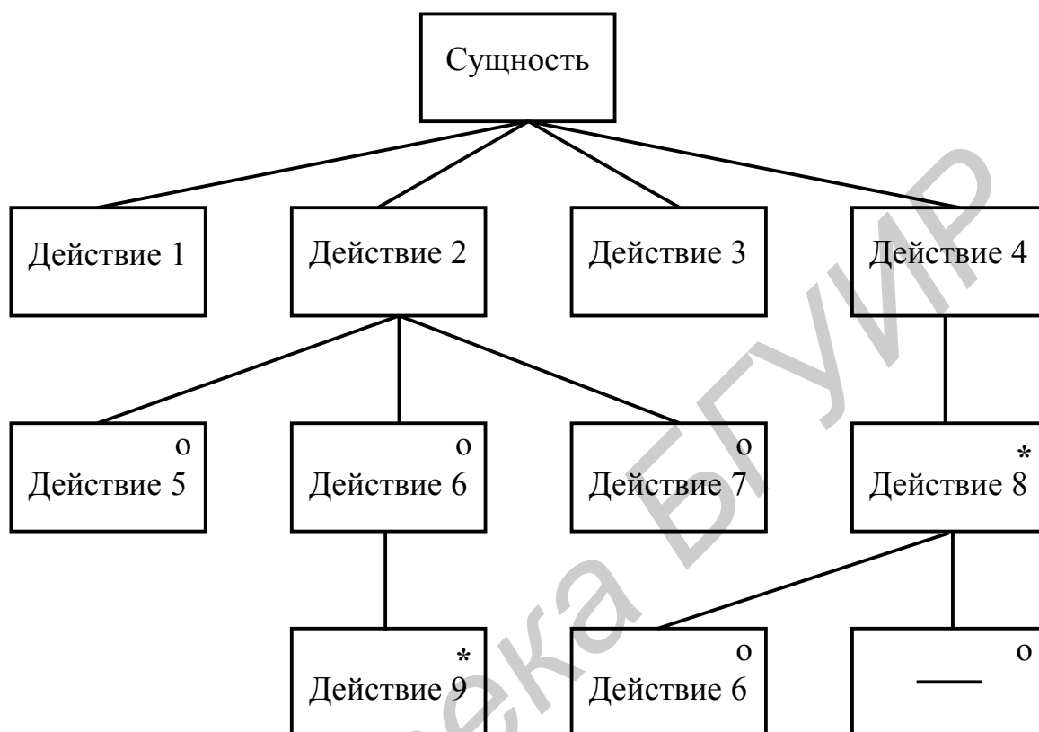
Рис. 5.49. Общий вид ESD-диаграммы
