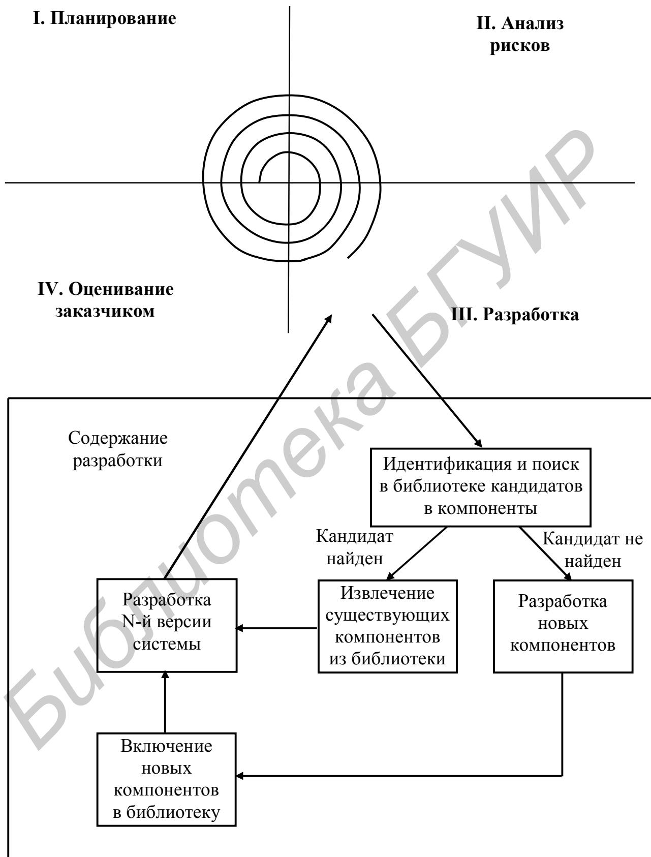
Рис. 2.23. Вариант компонентно-ориентированной спиральной модели
