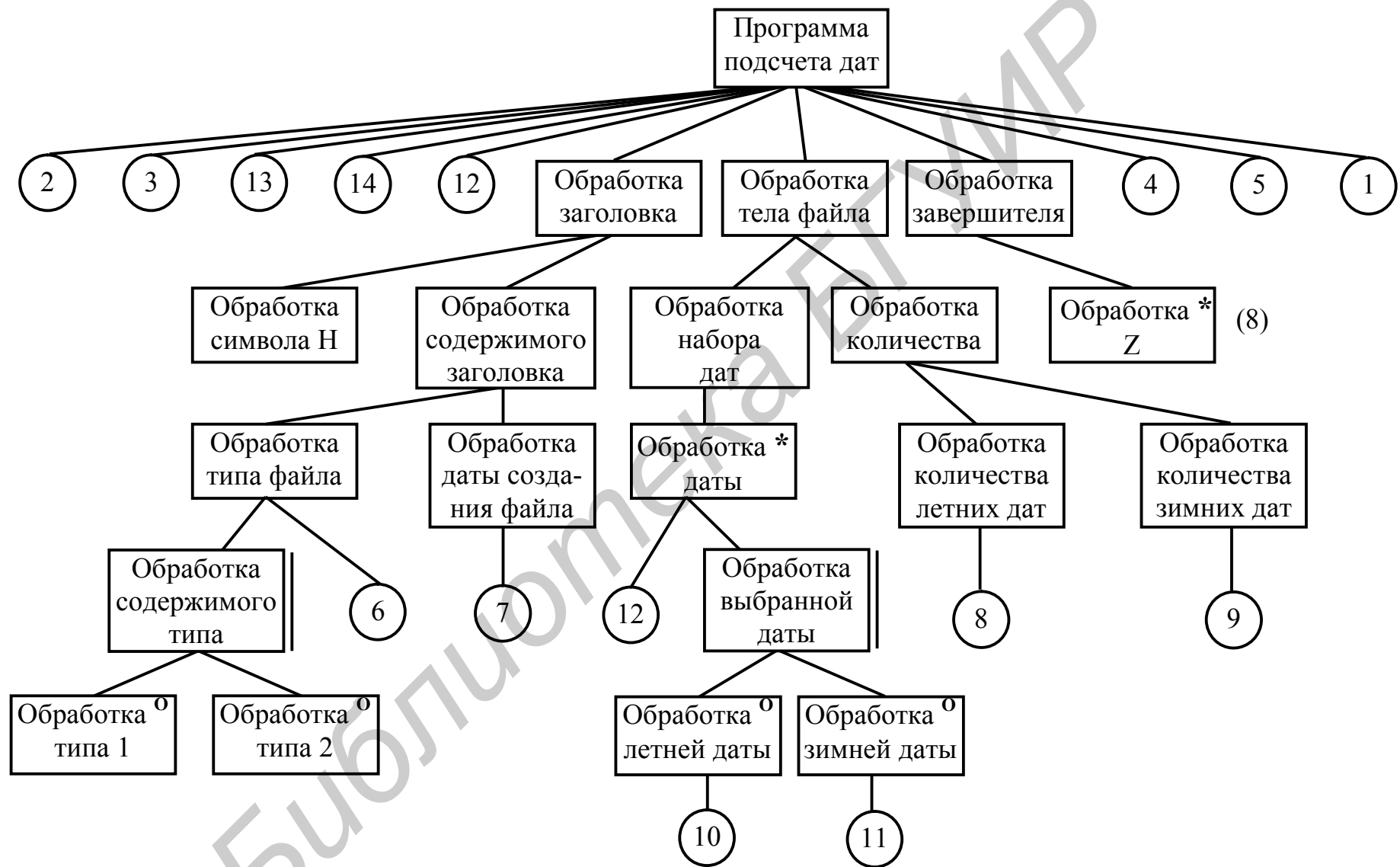
Рис. 4.55. Размещение выполняемых операций
