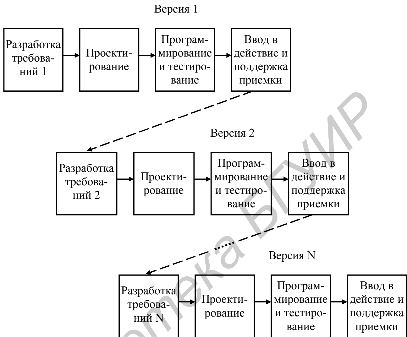
Рис. 2.15. Вариант эволюционной модели по ГОСТ Р ИСО/МЭК ТО 15271–2002
