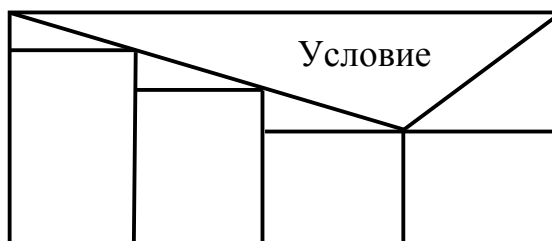
Рис. 4.17. Представление блока Case в схемах Насси–Шнейдермана
