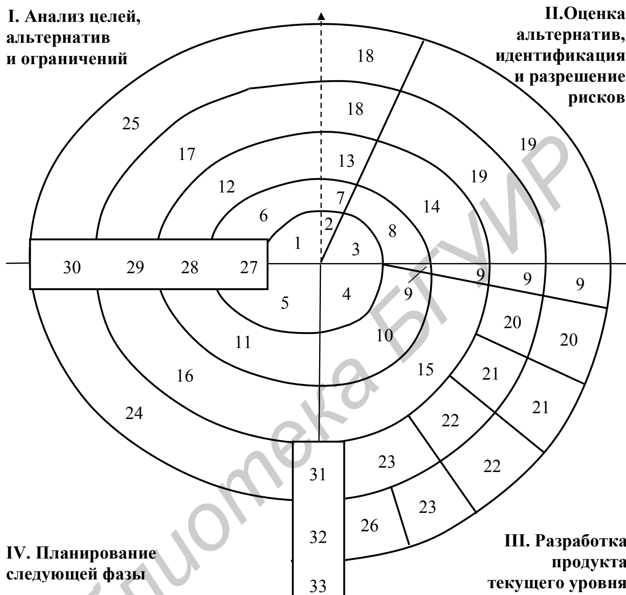
Рис. 2.18. Вариант спиральной модели Бозма, адаптированный к положениям стандарта СТБ ИСО/МЭК 12207–2003
