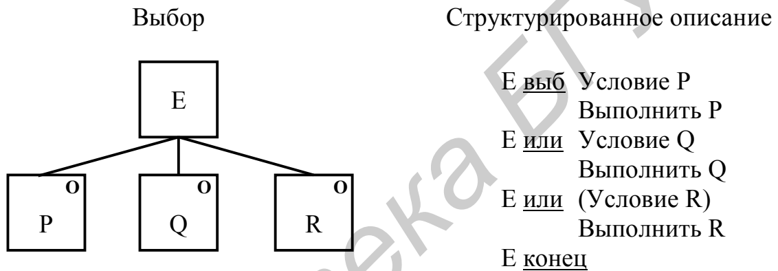
Рис. 4.57. Конструкция выбора и ее структурированное описание
