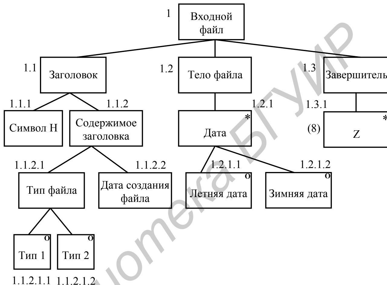
Рис. 4.49. Графическое представление структуры входного файла
