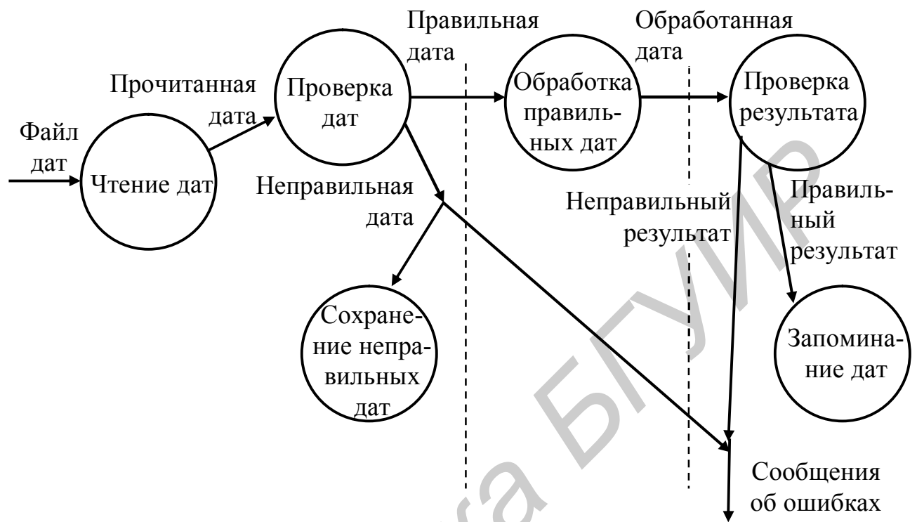
Рис. 4.22. Детализированная диаграмма потоков данных для программы обработки файла дат
