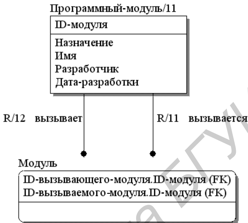
Рис. 5.40. Формализация рекурсивной связи мощностью многие-ко-многим посредством ассоциативной сущности
