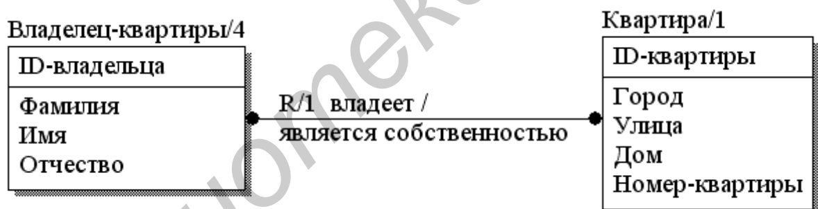
Рис. 5.34. Графическое представление в IDEF1X неспецифической связи
