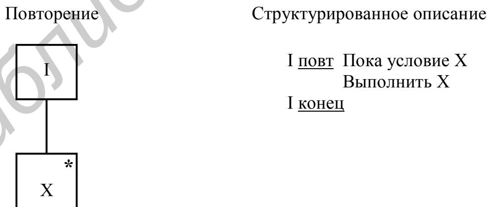
Рис. 4.58. Конструкция повторения и ее структурированное описание
