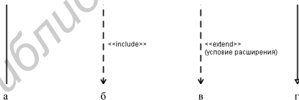
Рис. 6.4. Графическое представление отношений на диаграмме вариантов использования:
