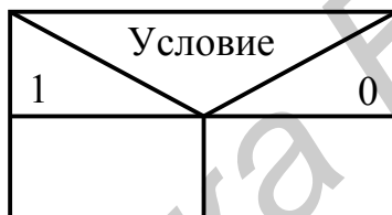
Рис. 4.16. Представление блока решения в схемах Насси–Шнейдермана
