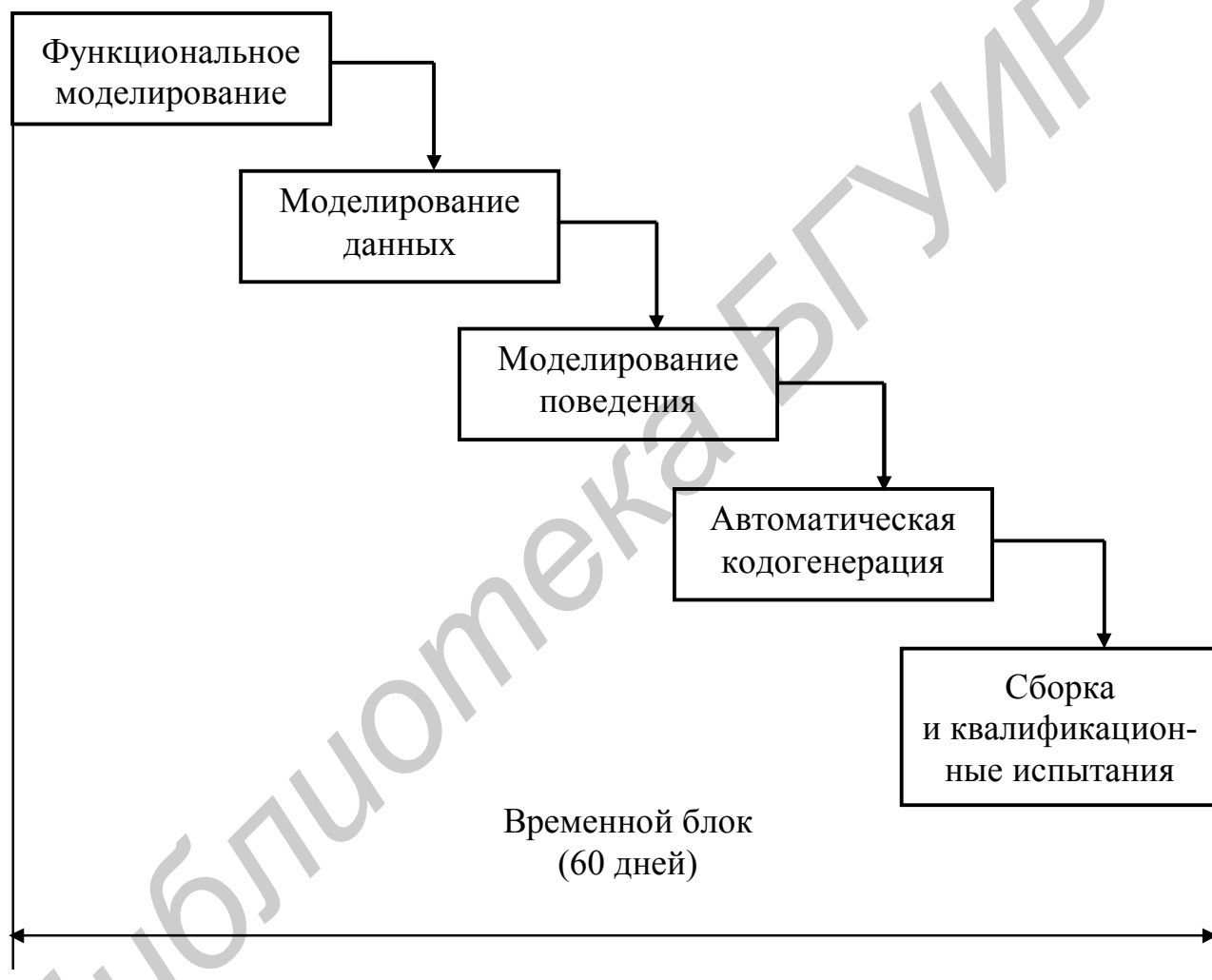
Рис. 2.9. Вариант модели быстрой разработки приложений, основанной на моделировании предметной области
