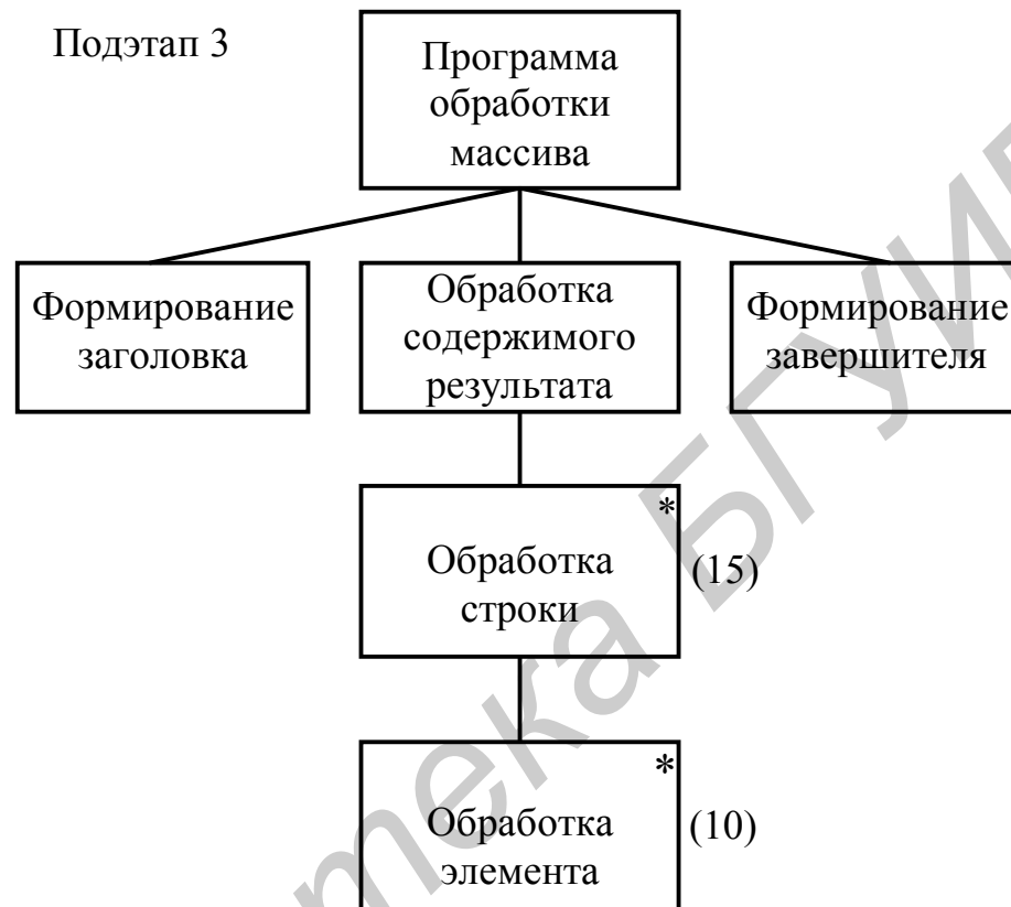
Рис. 4.48. Формирование полной структуры программы
