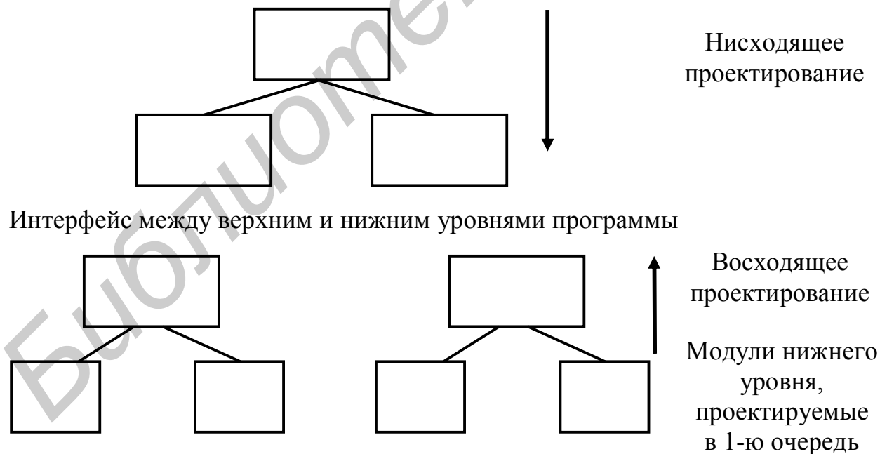
Рис. 4.28. Проектирование программы нисходящим и восходящим методами на базе модулей нижнего уровня
