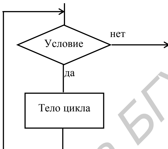
Рис. 4.3. Изображение конструкции обобщенного цикла в структурном программировании
