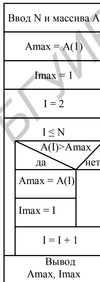
Детализированная схема Насси–Шнейдермана
