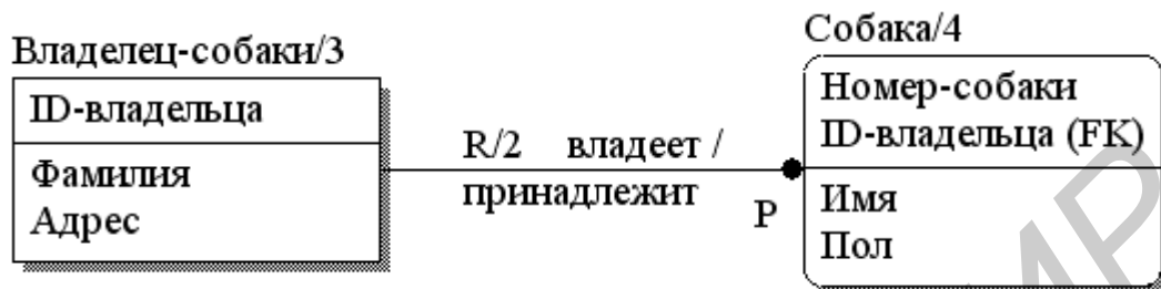
Рис. 5.25. Графическое представление в IDEF1X связи мощностью один-к-одному-или-многим
