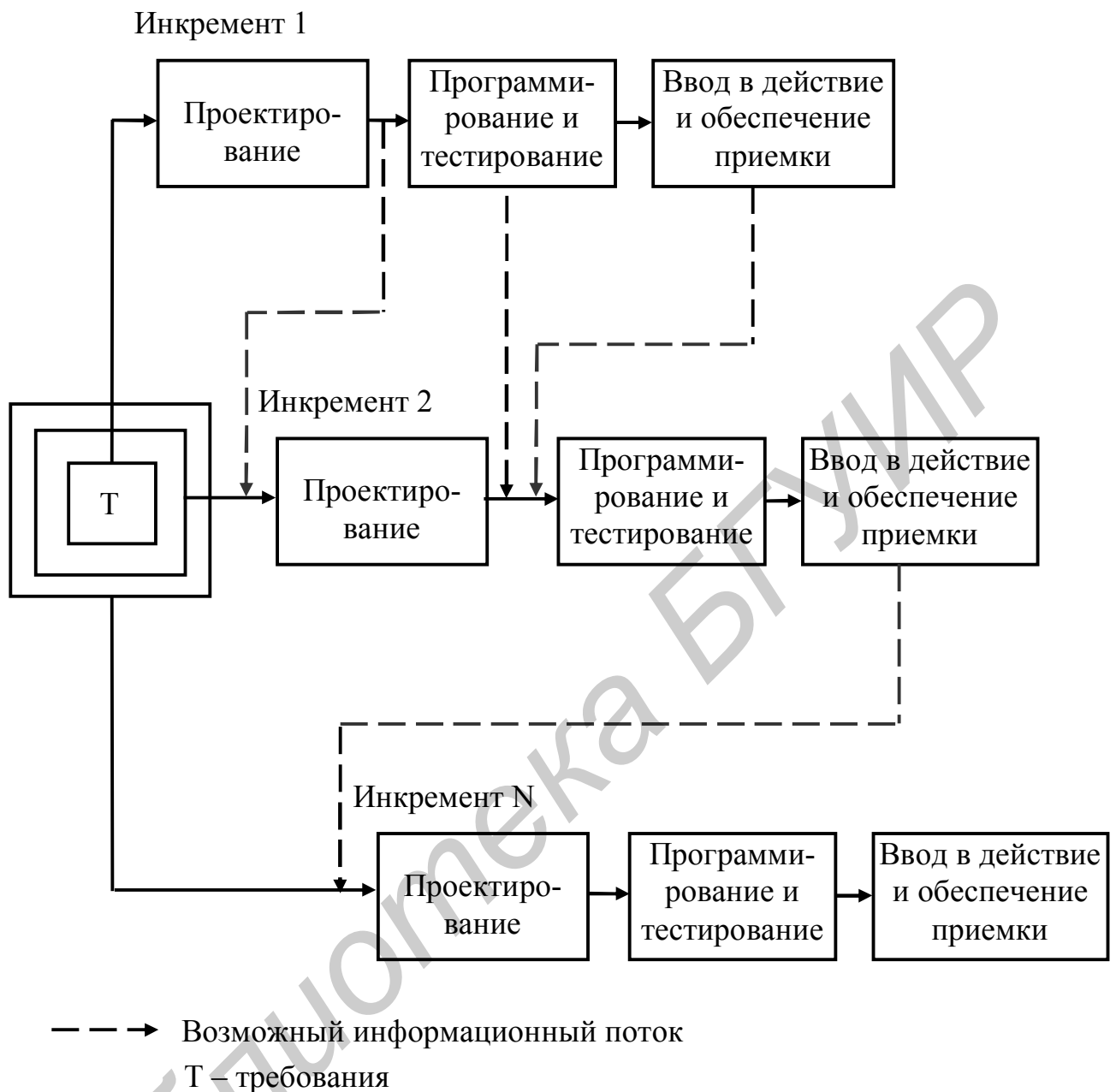
Рис. 2.13. Вариант инкрементной модели по ГОСТ Р ИСО/МЭК ТО 15271–2002
