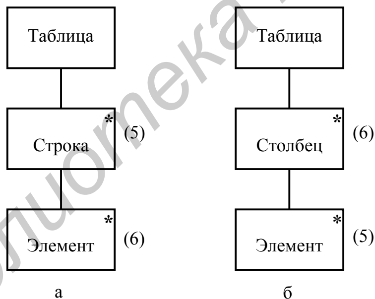
Рис. 4.41. Иерархическая структура таблиц: а – представление таблицы в виде набора строк; б – представление таблицы в виде набора столбцов
