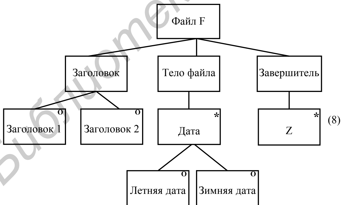
Рис. 4.37. Иерархическая структура данных
