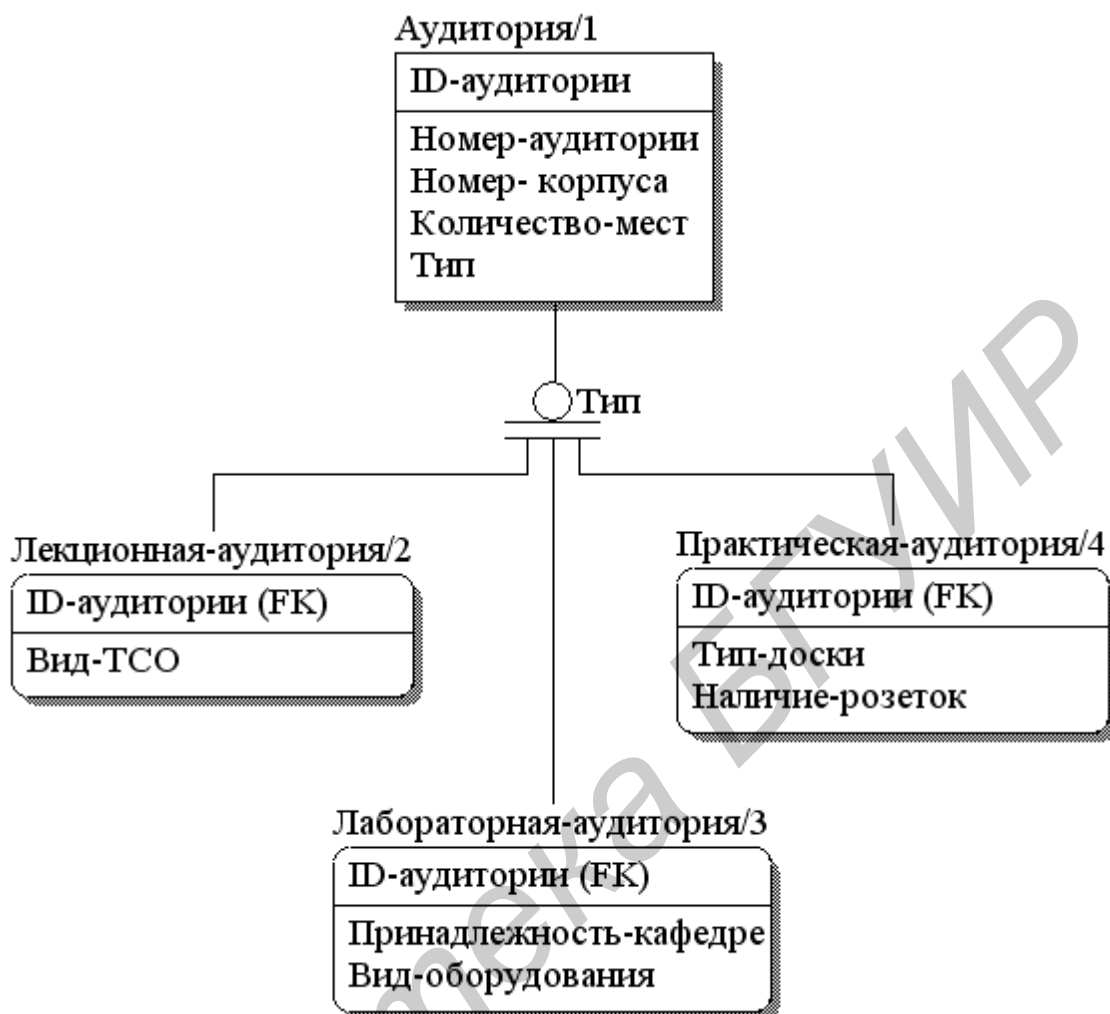
Рис. 5.43. Связь категоризации. Полная группа категорий
