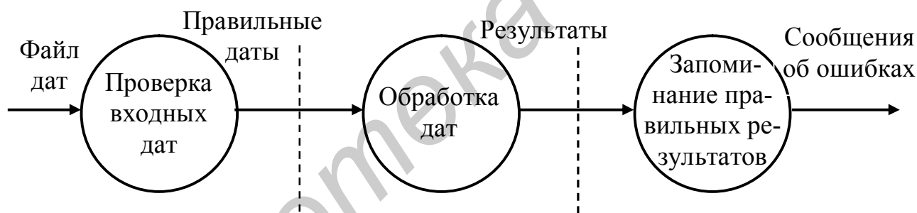
Рис. 4.21. Укрупненная диаграмма потоков данных для программы обработки файла дат
