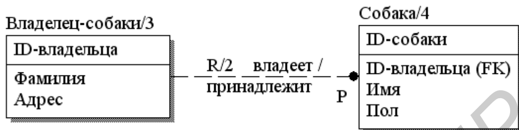
Рис. 5.30. Графическое представление в IDEF1X неидентифицирующей связи мощностью один-к-одному-или-многим
