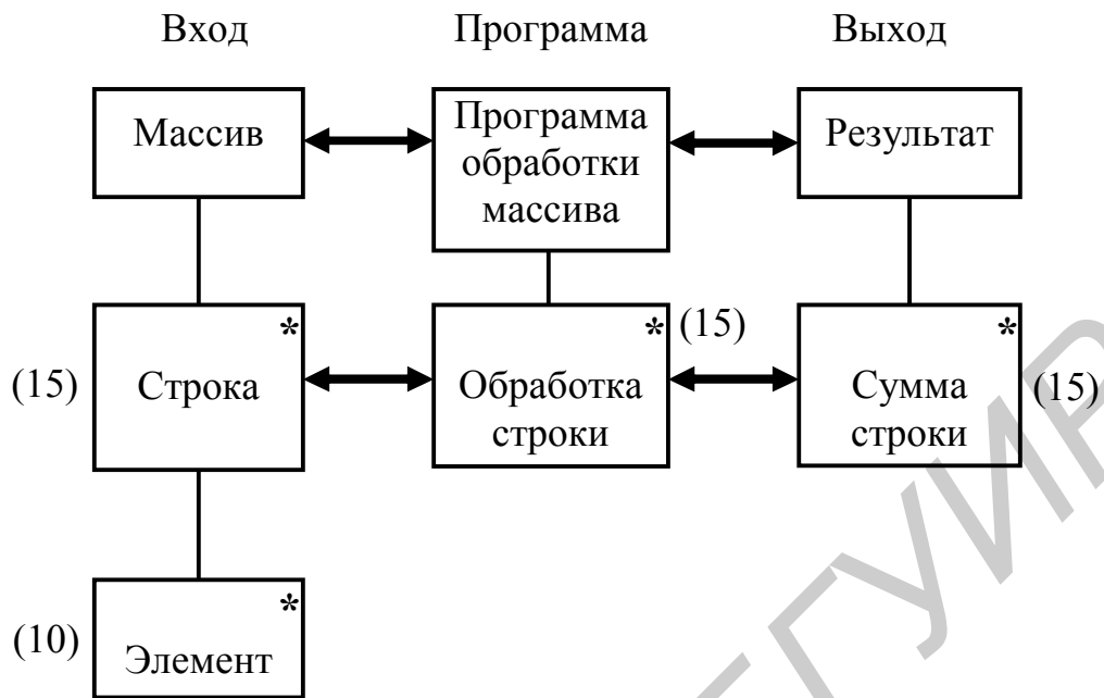
Рис. 4.44. Соответствие данных и программы
