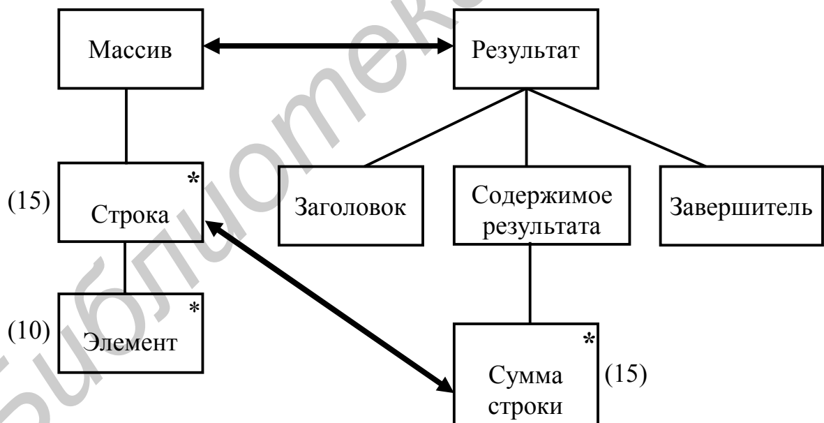
Рис. 4.45. Расширенные структуры входных и выходных данных
