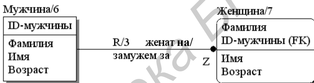
Рис. 5.26. Графическое представление в IDEF1X связи мощностью один-к-нулю-или-одному
