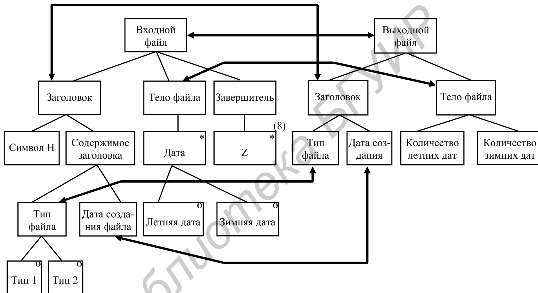
Рис. 4.51. Идентификация соответствий между входной и выходной структурами данных
