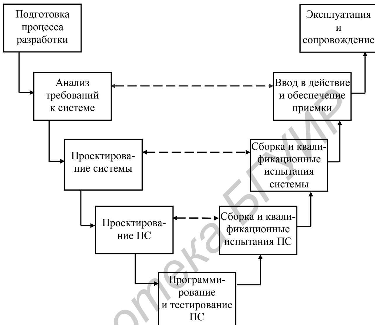
Рис. 2.6. V-образная модель жизненного цикла
