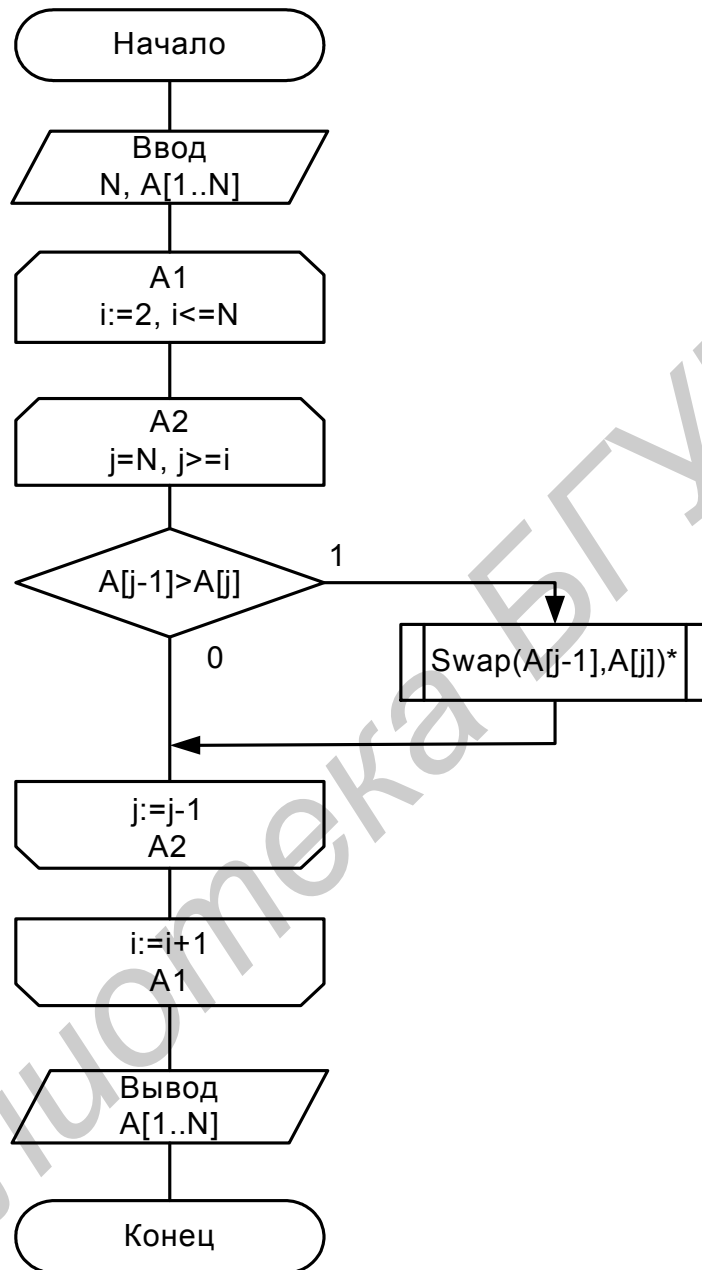
Схема алгоритма сортировки обменами (“пузырек”)
