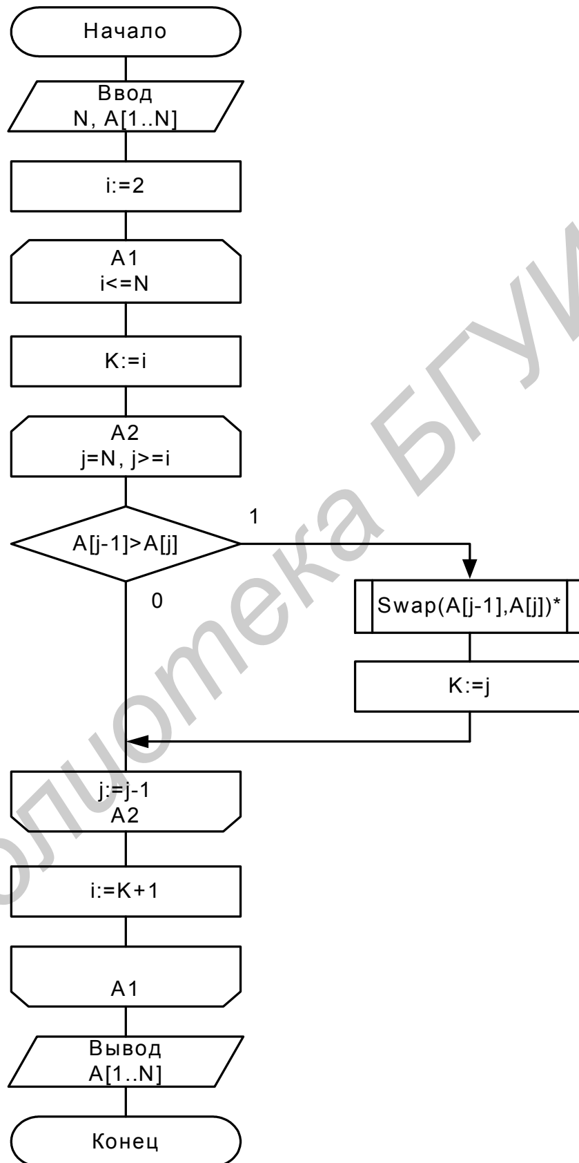
Схема алгоритма сортировки обменами с “быстрой границей”
